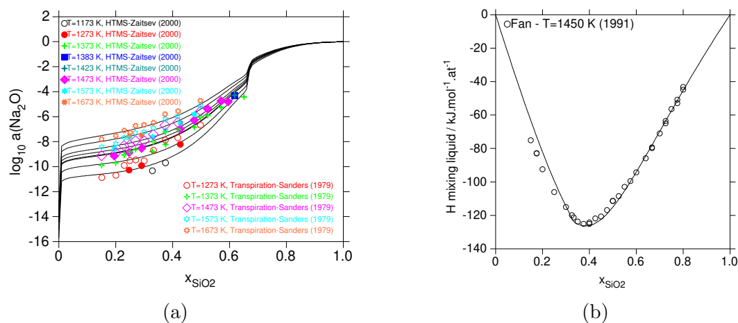
FIGURE 3.39 – (a) Activités de \text{Na}_2\text{O} à 1273 K, 1373 K, 1473 K, 1573 K et 1673 K, comparaison avec les mesures de Sanders & Haller [63] et de Zaitsev et al. [64], (b) Enthalpie de mélange du liquide \text{Na}_2\text{O}-\text{SiO}_2 à 1450 K, comparaison avec les mesures de Fan [65]
