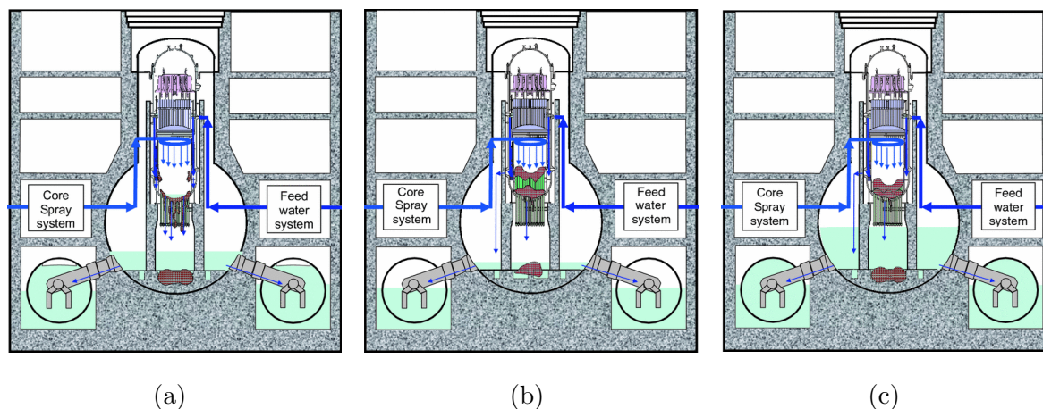
FIGURE D.2 – Estimation de la dégradation post-accidentelle des réacteurs de la centrale de Fukushima–Daïchi : (a) unité 1, (b) unité 2 : seul du liquide métallique est délocalisé, (c) unité 3 : des débris solides et liquides sont délocalisés
