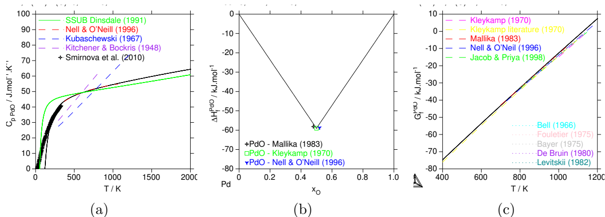
FIGURE C.13 – (a) Capacité calorifique de PdO, comparaison avec les données de la base SSUB [84], (b) Enthalpie de formation de PdO, (c) Enthalpie libre de formation de PdO
