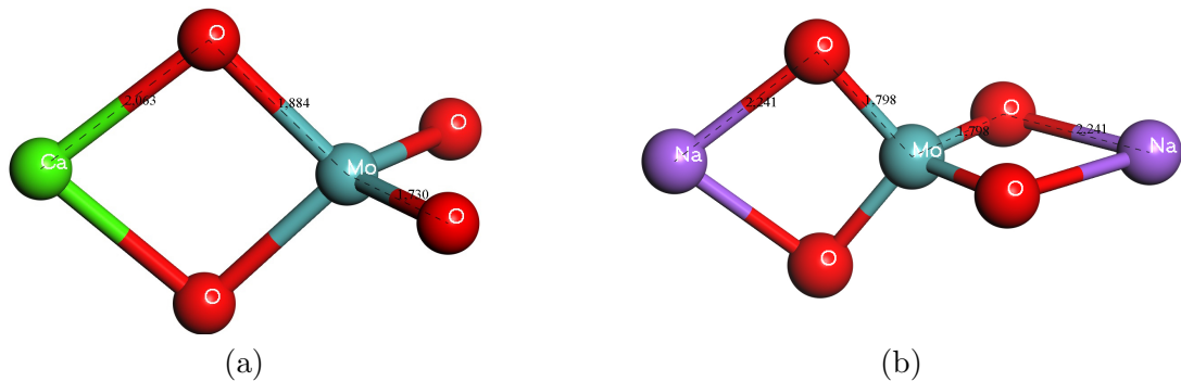
FIGURE 3.35 – Calculs DMol 3 de géométries à l'équilibre par J–L. Flèche de (a) \text{CaMoO}_4(\text{g}) de symétrie C_{2v} et (b) \text{Na}_2\text{MoO}_4(\text{g}) de symétrie D_{2d}
