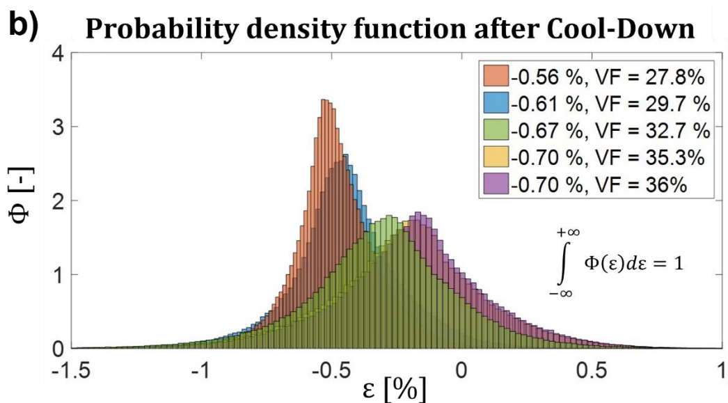
Figure 27. a) Carte des déformations simulées par MULTIFIL après CD pour deux VF différents ; b) Répartition des déformations après CD en fonction du VF (Riccioli 2020).
