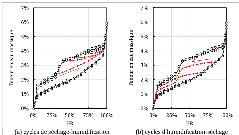
Figure 49 : mise en évidence du comportement hystérique d'un béton à 25°C avec la balance de sorption
