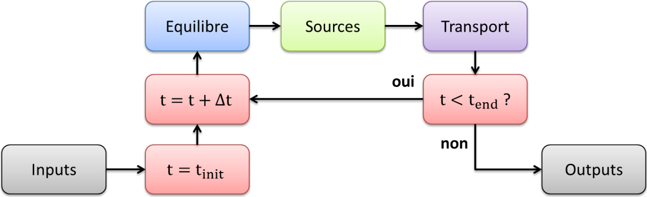
FIGURE 3.13: Schéma de la modélisation intégrée
