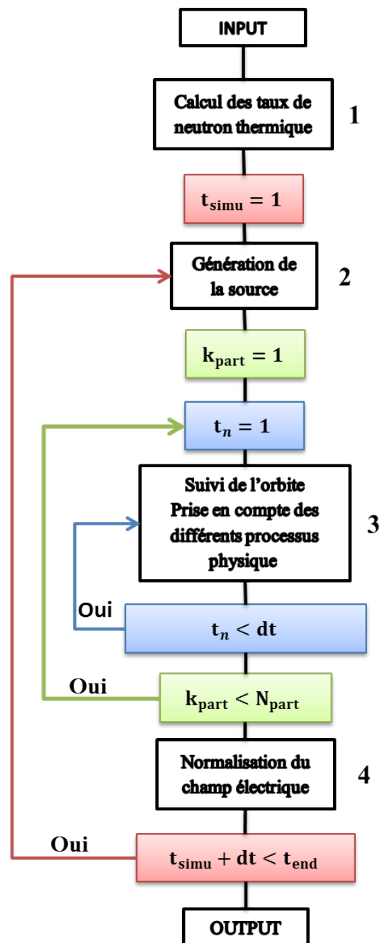
FIGURE 3.4: Représentation de la structure du code SPOT
