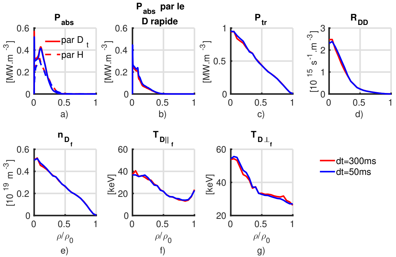
FIGURE 4.11: Comparaison des profils obtenus entre deux simulations auto-cohérentes EVE/SPOT, une dont le temps d'évolution de la distribution dt entre chaque itération est de 50ms (en bleu) et une autre où dt vaut 300ms (en rouge). a) Profils de la puissance ICRH absorbée par le D thermique et l'H. b) Profils de la puissance ICRH absorbée par le D rapide. c) Profils de la puissance transférée aux ions et électrons du plasma. d) Profils du taux de neutrons de la réaction D-D. e) Profils de la densité de D rapide. f) Profils de la température effective dans la direction parallèle du D rapide. g) Profils de la température effective dans la direction perpendiculaire du D rapide.
