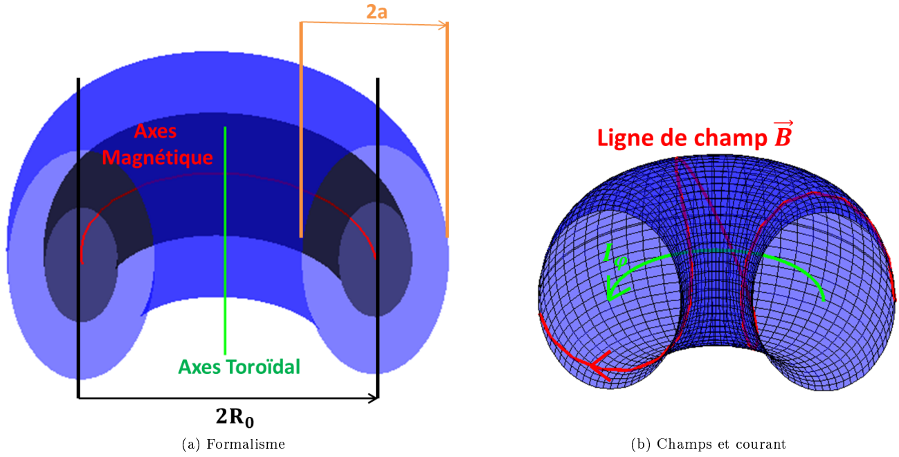
FIGURE 1.9: Principales caractéristiques d'un plasma de Tokamak
