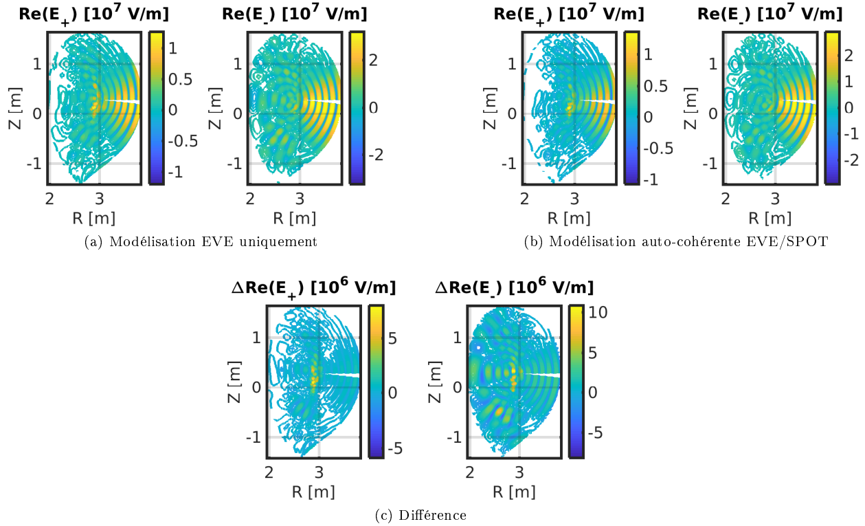
FIGURE 4.19: Comparaison de la partie réelle positive et négative du champ électrique de l'onde ICRF entre la simulation auto-cohérente EVE/SPOT (4.19b) et la simulation SPOT sans itération (4.19a) et la différence (4.19c).
