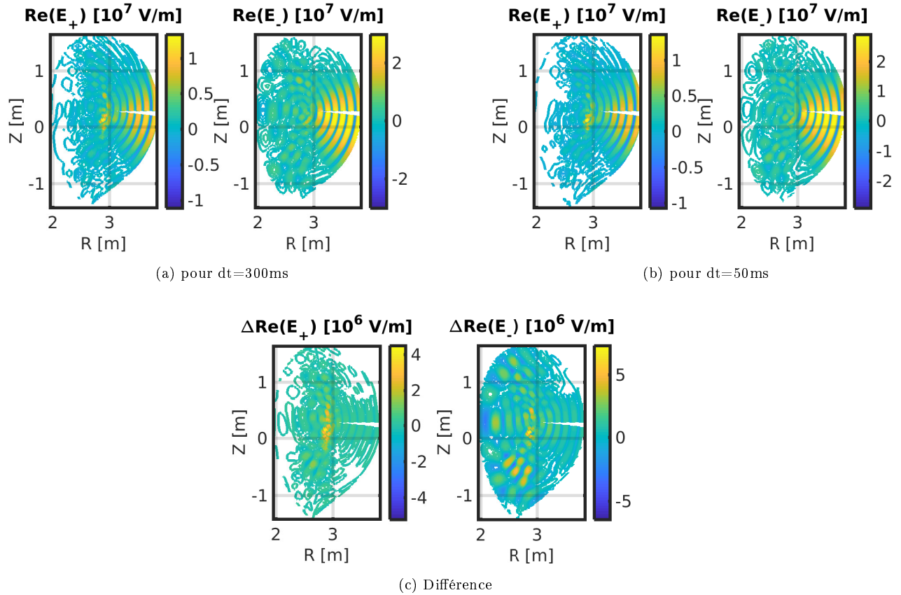
FIGURE 4.14: Comparaison de la partie réelle positive et négative du champ électrique de l'onde ICRF entre deux simulations auto-cohérentes EVE/SPOT, une dont le temps d'évolution de la distribution dt entre chaque itération est de 50ms (4.14b) et une autre où dt vaut 300ms (4.14a).
