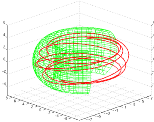
FIGURE 3.3: Représentation de la trajectoire 3D d'une particule piégée
