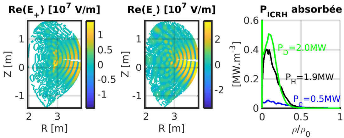
FIGURE 3.2: Exemple de la propagation et de l'absorption de l'onde ICRF pour un plasma de JET modélisé par EVE. De gauche à droite : Partie réelle de la composante positive et négative du champ électrique de l'onde ICRF représentant sa polarisation, profils de la puissance ICRH absorbée par l'hydrogène (en noir), le deutérium (en vert) et les électrons (en bleu) avec les valeurs des puissances absorbées intégrées sur le volume plasma.
