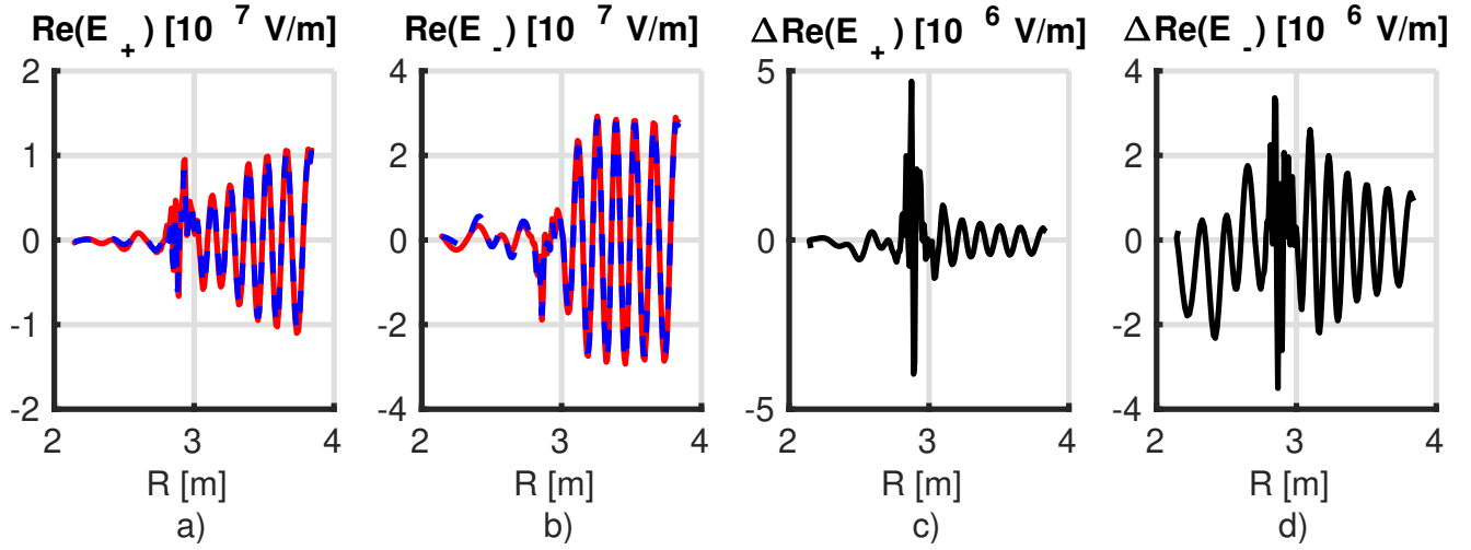
FIGURE 4.13: Comparaison de la partie réelle positive (a) et négative (b) de la composante électrique de l'onde ICRF entre deux simulations auto-cohérentes EVE/SPOT, une dont le temps d'évolution de la distribution dt entre chaque itération est de 50ms (en bleu) et une autre où dt vaut 300ms (en rouge), dans la plan équatorial. Différence de la composante positive (c) et négative (d) du champ électrique de l'onde ICRF entre les deux modélisations.
