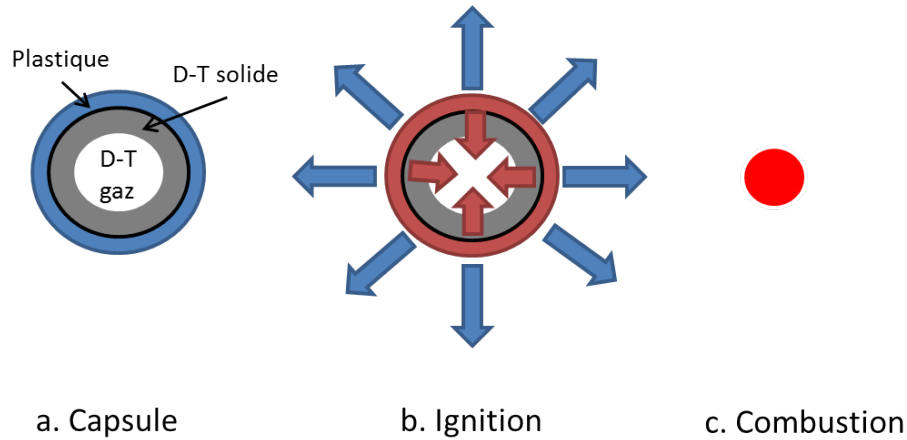
FIGURE 1.4: Schéma du processus de fusion inertielle
