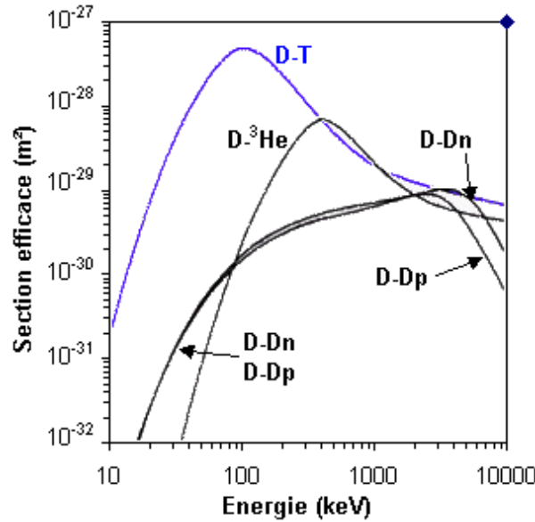
FIGURE 1.2: Sections efficaces des différentes réactions de fusion en fonction de l'énergie des réactants [2]
