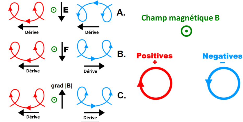
FIGURE 1.11: Illustration des vitesses de dérive électromagnétique pour les ions (en rouge) et électrons (en bleu). La configuration A illustre la vitesse de dérive \vec{E} \wedge \vec{B} , la configuration B illustre une vitesse de dérive due à une force \vec{F} et la configuration C illustre la vitesse de dérive due au gradient du champ magnétique.
