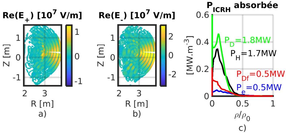
FIGURE 4.7: Partie réelle de la composante positive (a) et négative (b) du champ électrique de l'onde ICRF. c) Profils de la puissance ICRH absorbée par l'hydrogène (en noir), le deutérium thermique (en vert), le deutérium rapide (en rouge) et les électrons (en bleu) avec les valeurs des puissances absorbées intégrées sur le volume plasma.
