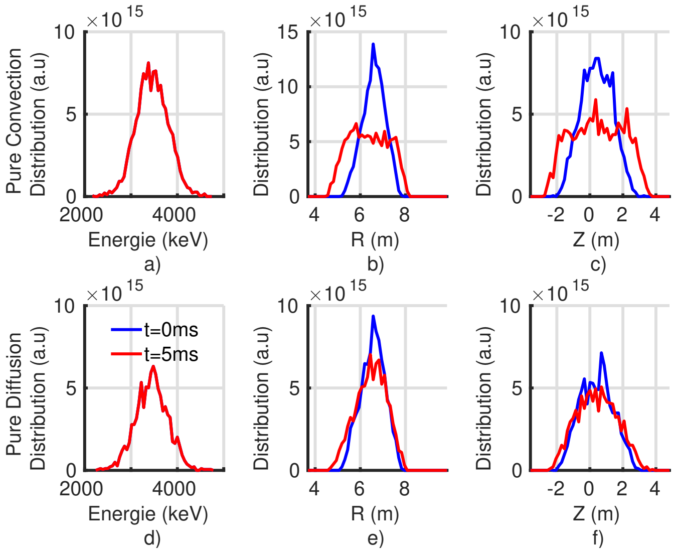
FIGURE 3.7: Impact du transport anormal sur la distribution des particules
