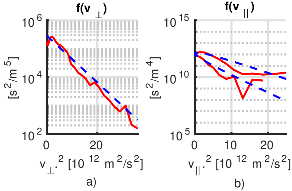
FIGURE 4.8: Comparaison de la distribution de SPOT f_S à l'état stationnaire (cf eq.4.1 et eq.4.2) (en rouge) avec le fit bi-maxwellien f_F (cf eq.4.3 et eq.4.4) (en tiret bleu) à \rho/\rho_0 = 0.1 .
