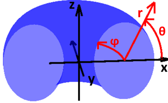
FIGURE 1.8: Coordonnées cartésiennes (en noir) et coordonnées curvilignes toroïdales (en rouge) des plasmas de Tokamak (en bleu)
