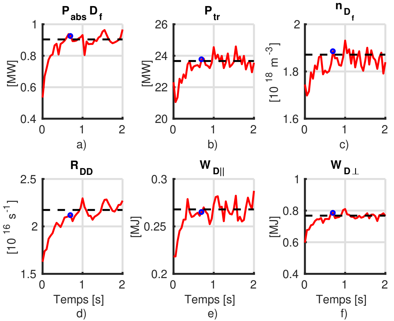
FIGURE 4.9: Évolution des quantités globales du plasma de la simulation itérative EVE/SPOT avec 2% d'H et une évolution de 50ms de la distribution entre chaque itération. a) Evolution de la puissance ICRH absorbée par le D rapide. b) Evolution de la puissance transférée au plasma. c) Evolution de la densité de D rapide. d) Evolution du taux de neutrons de la réaction D-D. e) Evolution du contenu énergétique dans la direction parallèle. f) Evolution du contenu énergétique dans la direction perpendiculaire.
