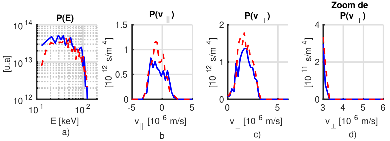
FIGURE 4.21: Comparaison de la distribution énergétique (a), de la distribution en vitesse parallèle (b) et de la distribution en vitesse perpendiculaire (c et d) du D rapide à \rho/\rho_0 = 0.1 obtenus par NEMO/SPOT avec différents profils d'input de T_i .
