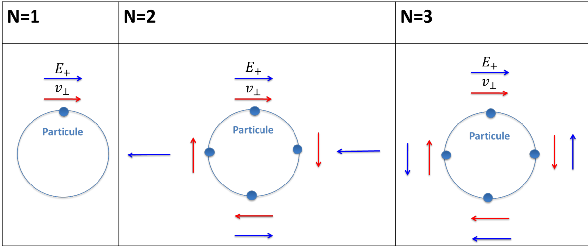
FIGURE 1.13: Schéma de la polarisation de l'onde avec la pulsation cyclotronique en fonction de l'harmonique
