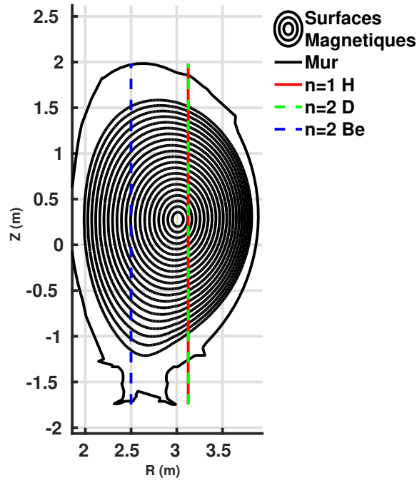
FIGURE 4.1: Coupe poloïdale du mur, des surfaces magnétiques et des couches de résonances du chauffage ICRH à la fréquence \omega = 42.5 MHz
