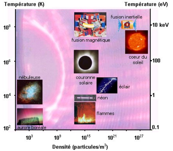
FIGURE 1.3: Classification des différents plasmas en fonction de la densité et de la température [3]
