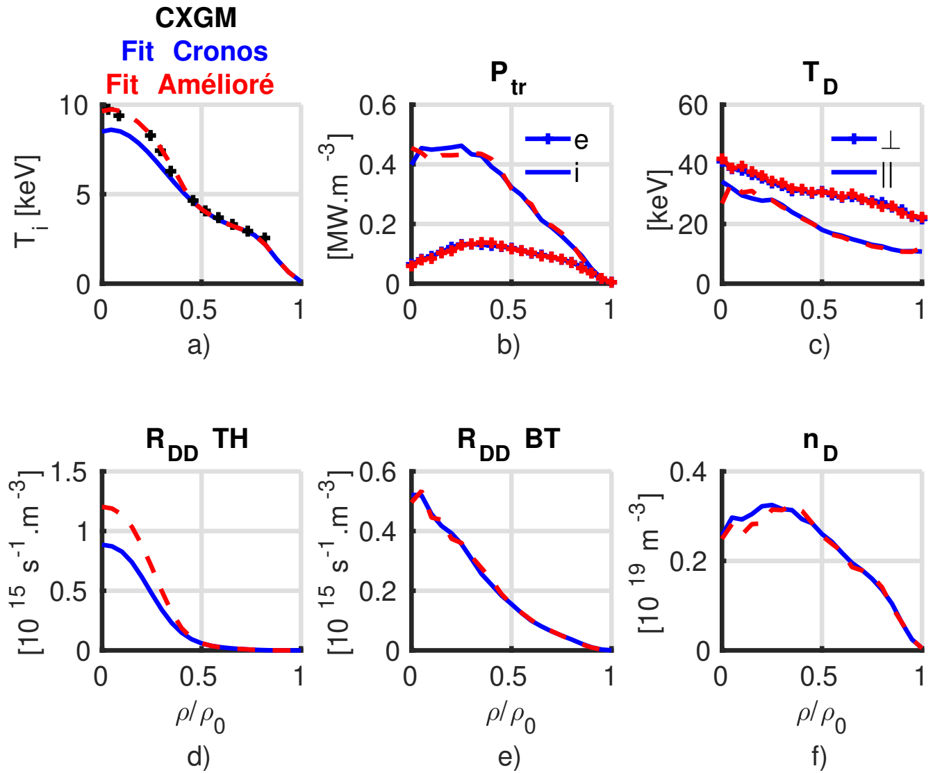
FIGURE 4.20: Comparaison des profils obtenus par les modélisations NEMO/SPOT pour différents profils d'input de T_i . a) Profils d'input de T_i . b) Profils de la puissance transférée aux ions et électrons du plasma. c) Profils des températures effectives perpendiculaire et parallèle. d) Profils des taux de neutrons des réactions thermiques. e) Profils des taux de neutrons des réactions beam-target. f) Profils de la densité de D rapide.
