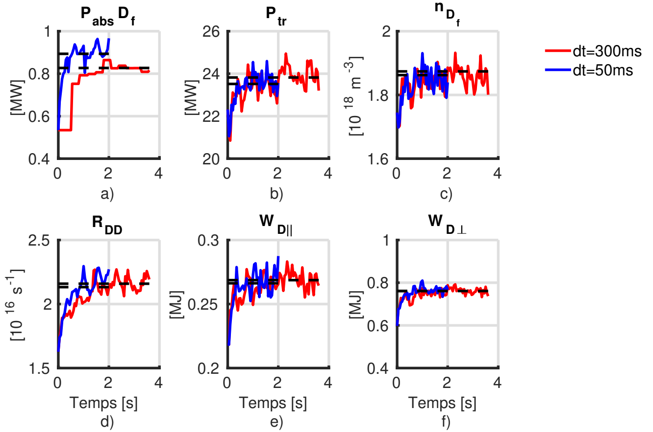
FIGURE 4.10: Comparaison de l'évolution des quantités globales du plasma entre deux simulations auto-cohérentes EVE/SPOT, une dont le temps d'évolution de la distribution dt entre chaque itération est de 50ms (en bleu) et une autre où dt vaut 300ms (en rouge). a) Évolution de la puissance ICRH absorbée par le D rapide. b) Évolution de la puissance transférée aux ions et électrons du plasma. c) Évolution de la densité du D rapide. d) Évolution du taux de neutrons de la réaction D-D. e) Evolution du contenu énergétique dans la direction parallèle. f) Évolution du contenu énergétique dans la direction perpendiculaire.
