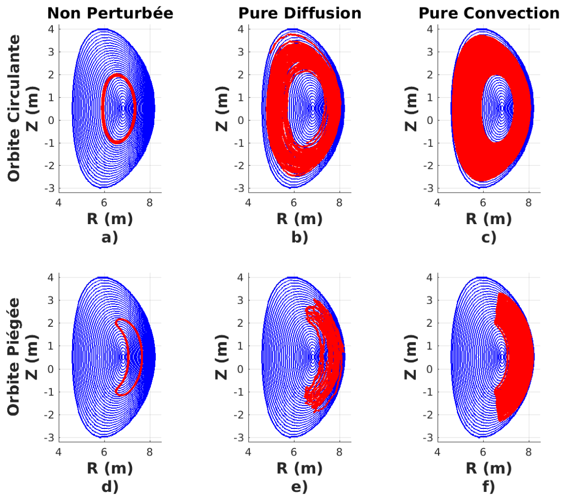
FIGURE 3.6: Impact du transport anormal sur les orbites des particules
