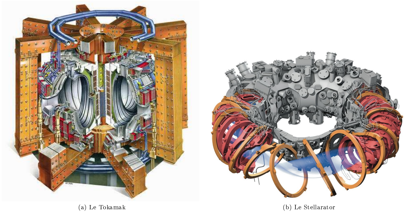
FIGURE 1.7: Image en coupe des dispositifs pour réaliser la fusion nucléaire.
