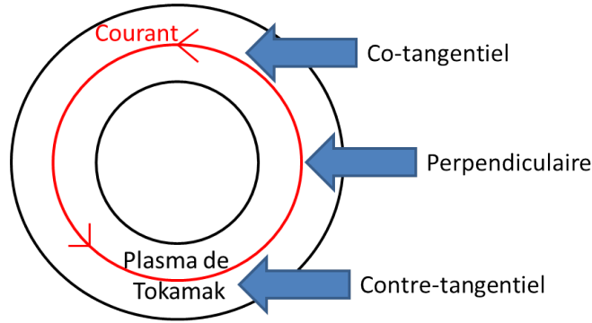
FIGURE 2.3: Schéma des différentes géométries d'injection du chauffage NBI, vues du dessus
