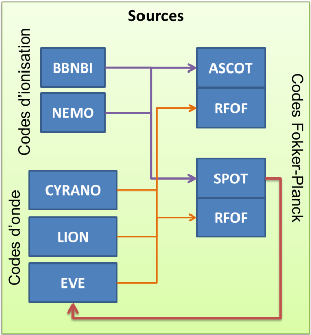
FIGURE 3.14: Schéma de la diversité et flexibilité des codes de la plateforme EUTM pour la modélisation des chauffages ioniques
