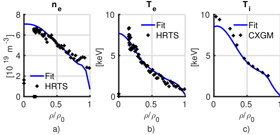
FIGURE 4.2: Comparaison des profils de densité (a) et de température (b) électronique et de température ionique (c) entre le fit provenant de CRONOS (en bleu) et les données expérimentales de JET (en symboles noir) du choc #86614.
