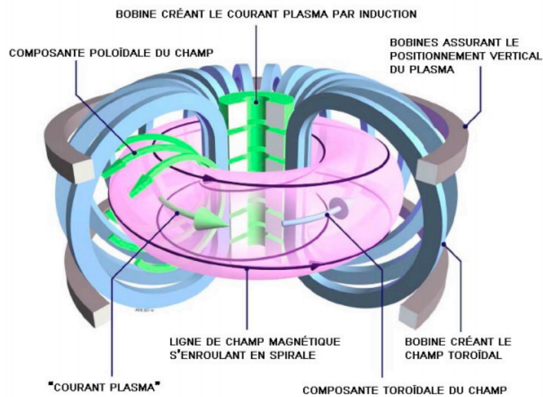
FIGURE 1.6: Schéma de la mécanique de la configuration fermée [5]
