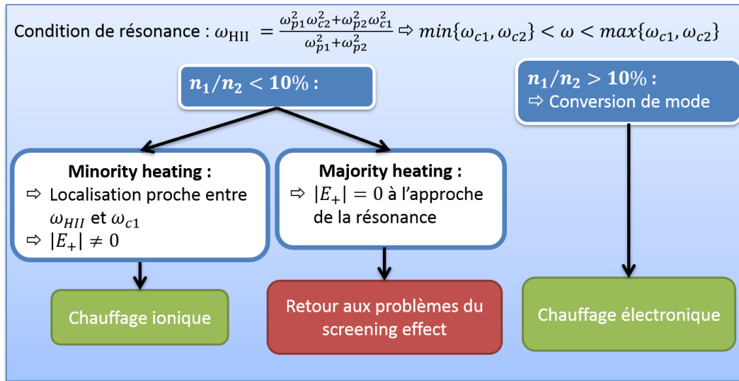
FIGURE 2.6: Schéma récapitulatif du scénario de chauffage ICRH pour un plasma composé de deux espèces ioniques
