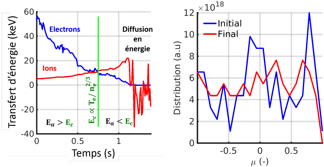
(a) Transfert énergétique de la particule alpha sur les ions (en rouge) et sur les électrons (en bleu) du plasma (b) Distribution des particules alpha en fonction du pitch angle pour l'état initial (en bleu) et final (en rouge)
