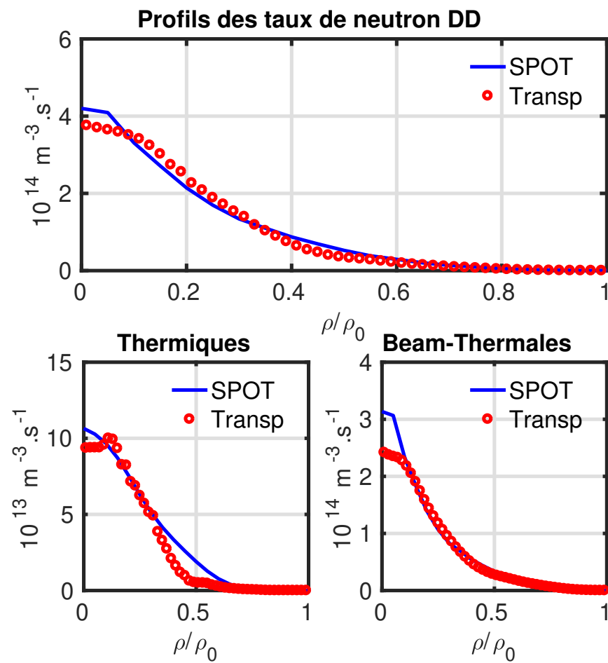
FIGURE 3.10: Comparaison des profils des taux de neutrons obtenus par la modélisation de SPOT (en bleu) et par celle de TRANSP (en rouge) de la décharge 84792 de JET
