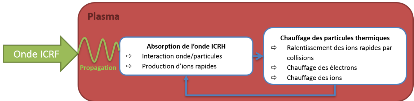
FIGURE 2.5: Schéma conceptuel du chauffage plasma par l'onde ICRF
