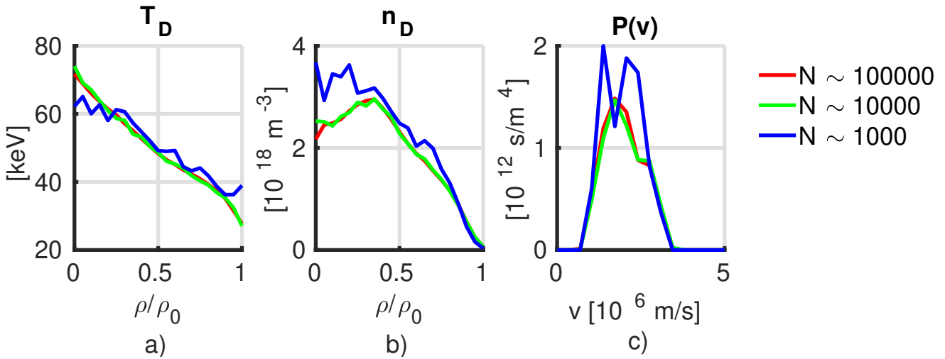
FIGURE 4.4: Comparaison des profils de température (a) et de densité (b) du D rapide et de la distribution Monte-Carlo donnée par SPOT à \rho/\rho_0 = 0.1 (c) pour trois valeurs du nombre de particule N : N \sim 100000 (en rouge), N \sim 10000 (en vert), N \sim 1000 (en bleu).
