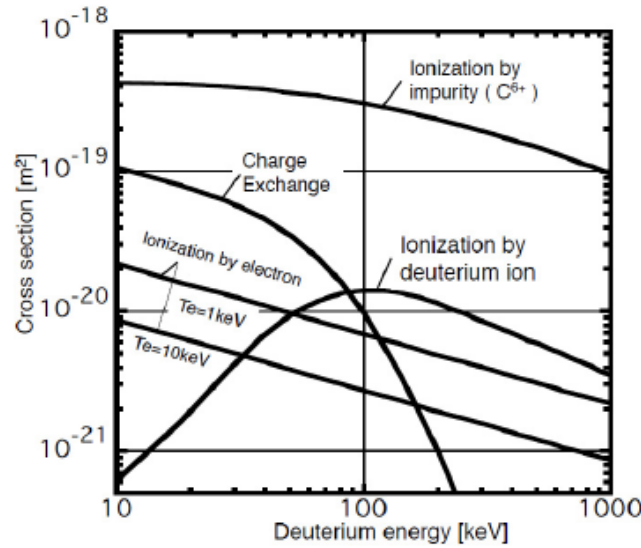
FIGURE 2.4: Dépendance des différentes sections efficaces en fonction de l'énergie du faisceau [8]
