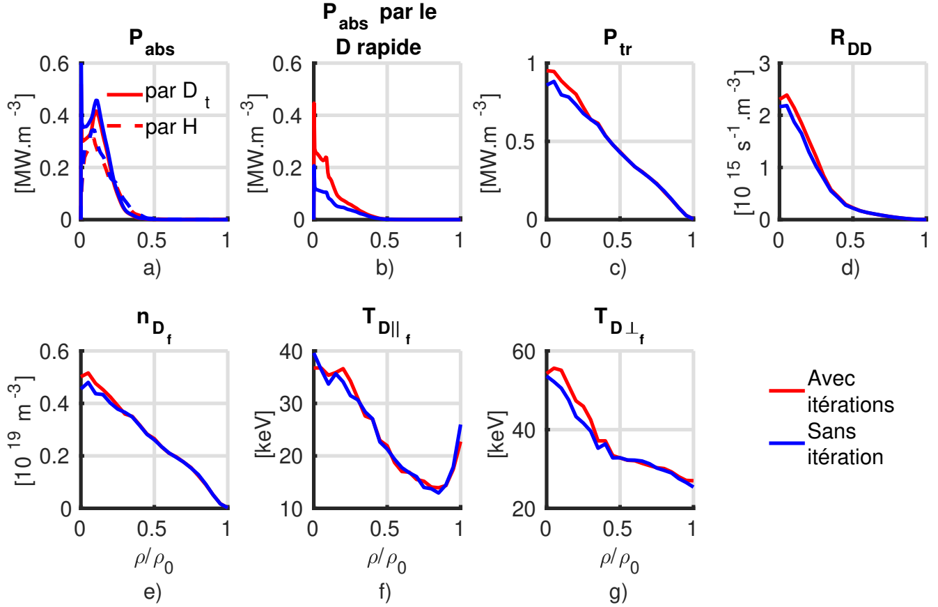
FIGURE 4.16: Comparaison des profils obtenus par la simulation auto-cohérente EVE/SPOT (en rouge) et la simulation SPOT sans itération (en bleu). a) Profils de la puissance ICRH absorbée par le D thermique et l'H. b) Profils de la puissance ICRH absorbée par le D rapide. c) Profils de la puissance transférée aux ions et électrons du plasma. d) Profils du taux de neutrons de la réaction D-D. e) Profils de la densité de D rapide. f) Profils de la température effective dans la direction parallèle du D rapide. g) Profils de la température effective dans la direction perpendiculaire du D rapide.
