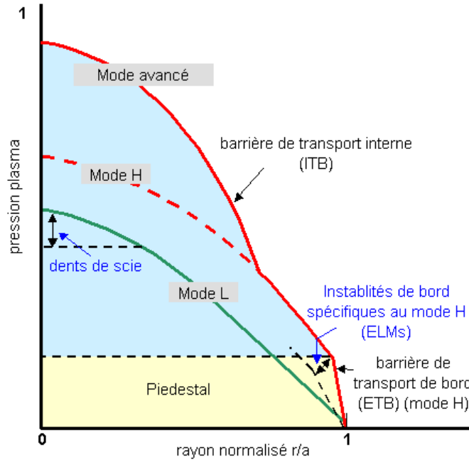
FIGURE 1.10: Profils de pression associés aux différents mode de confinement [6]
