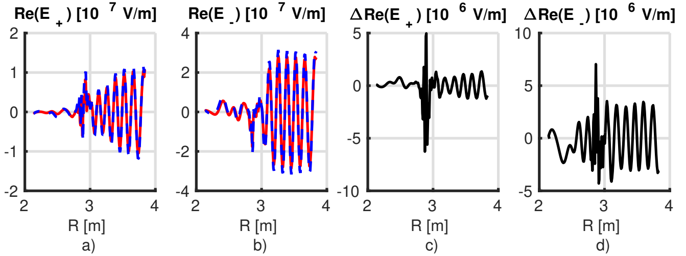
FIGURE 4.18: Comparaison de la partie réelle positive (a) et négative (b) de la composante électrique de l'onde ICRF entre la simulation auto-cohérente EVE/SPOT (en rouge) et la simulation SPOT sans itération (en bleu) dans la plan équatorial. Différence de la composante positive (c) et négative (d) du champ électrique de l'onde ICRF entre les deux modélisations.
