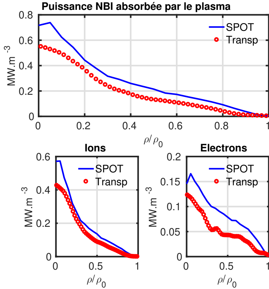
FIGURE 3.11: Comparaison des profils de la puissance NBI absorbée par le plasma obtenus par la modélisation de SPOT (en bleu) et par celle de TRANSP (en rouge) de la décharge 84792 de JET
