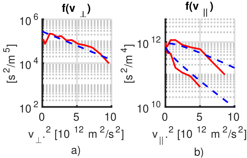
FIGURE 4.6: Comparaison de la distribution de SPOT f_S (cf eq.4.1 et eq.4.2) (en rouge) avec le fit bi-maxwellien f_F (cf eq.4.3 et eq.4.4) (en tiret bleu) à \rho/\rho_0 = 0.1 .
