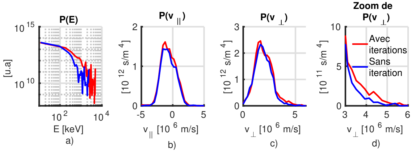
FIGURE 4.17: Comparaison de la distribution énergétique (a), de la distribution en vitesse parallèle (b) et perpendiculaire (c et d) du D rapide à \rho/\rho_0 = 0.1 entre la simulation auto-cohérente EVE/SPOT (en rouge) et la simulation SPOT sans itération (en bleu).
