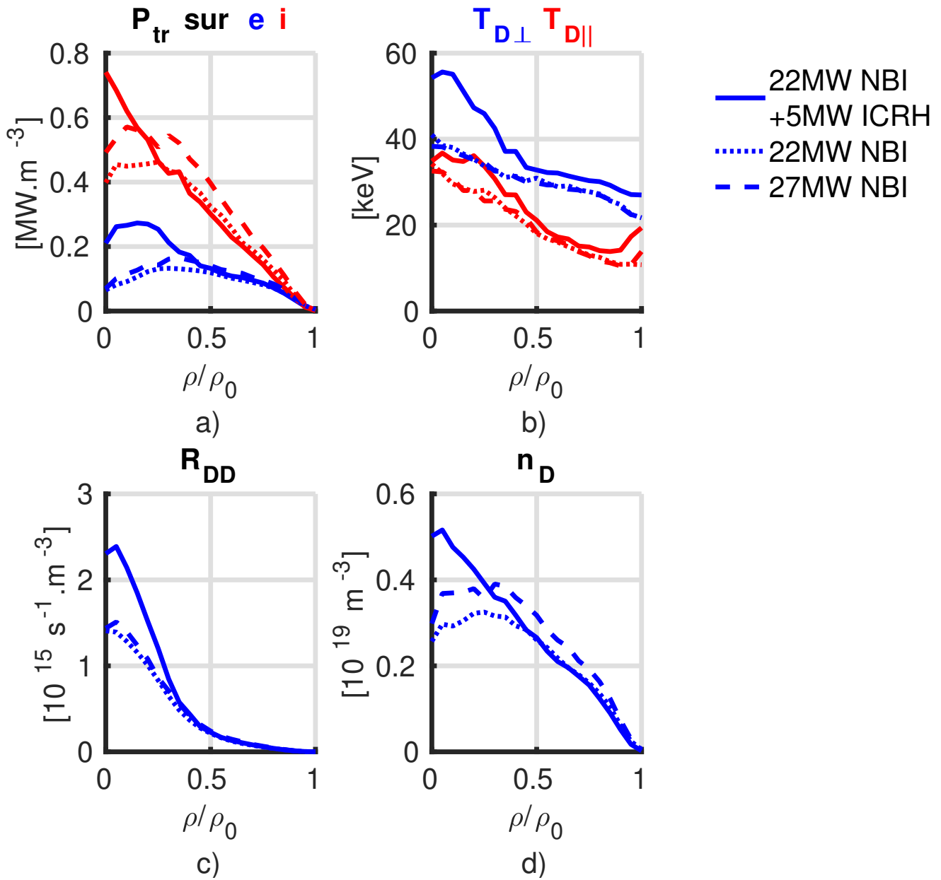
FIGURE 4.22: Comparaison des profils obtenus par la modélisation avec 27MW de puissance NBI (en tiret), la modélisation avec 22MW de puissance NBI et 5MW d'ICRH (en ligne pleine) et la modélisation avec 22MW de puissance NBI (en pointillés). a) Profils de la puissance transférée aux ions (en rouge) et électrons (en bleu) du plasma. b) Profils des températures effectives perpendiculaire (en bleu) et parallèle (en rouge). c) Profils des taux de neutrons de la réaction D-D. d) Profils de la densité de D rapide.
