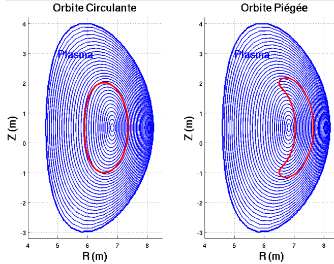
FIGURE 1.12: Projection dans une section poloïdale de la trajectoire des particules passantes (ou orbites circulantes) et des particules piégées (ou orbites banane) modélisée par SPOT.
