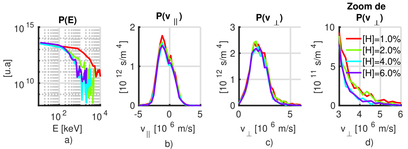
FIGURE 4.26: a) Comparaison de la distribution énergétique du D rapide pour différentes concentrations d'H (1%, 2%, 4%, 6%) à \rho/\rho_0 = 0.1 . b) Comparaison de la distribution des vitesses parallèles du D rapide pour différentes concentrations d'H (1%, 2%, 4%, 6%) à \rho/\rho_0 = 0.1 . c) et d) Comparaison de la distribution des vitesses perpendiculaires du D rapide pour différentes concentrations d'H (1%, 2%, 4%, 6%) à \rho/\rho_0 = 0.1 .
