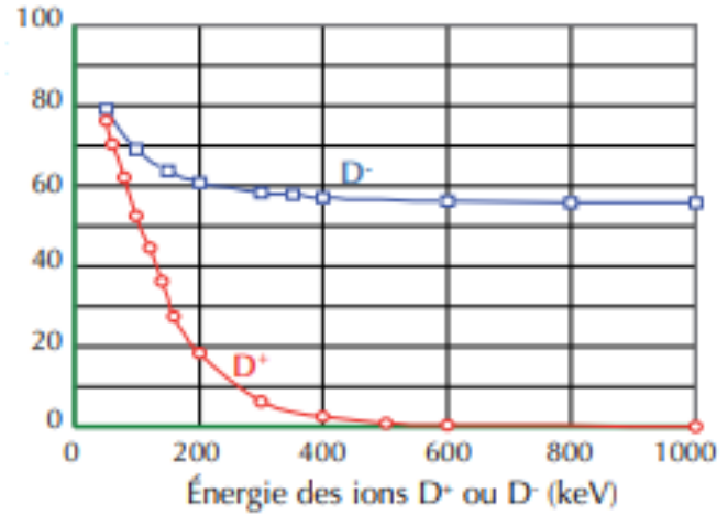
FIGURE 2.2: Taux de neutralisation des ions D^+ et D^- en fonction de leur énergie. [7]
