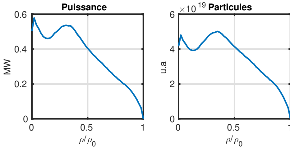
FIGURE 3.1: Exemple de profils de déposition 1D de puissance et de particules produit par le système NBI de JET pour une puissance de 22MW dans un plasma de D (#86614) modélisé par NEMO
