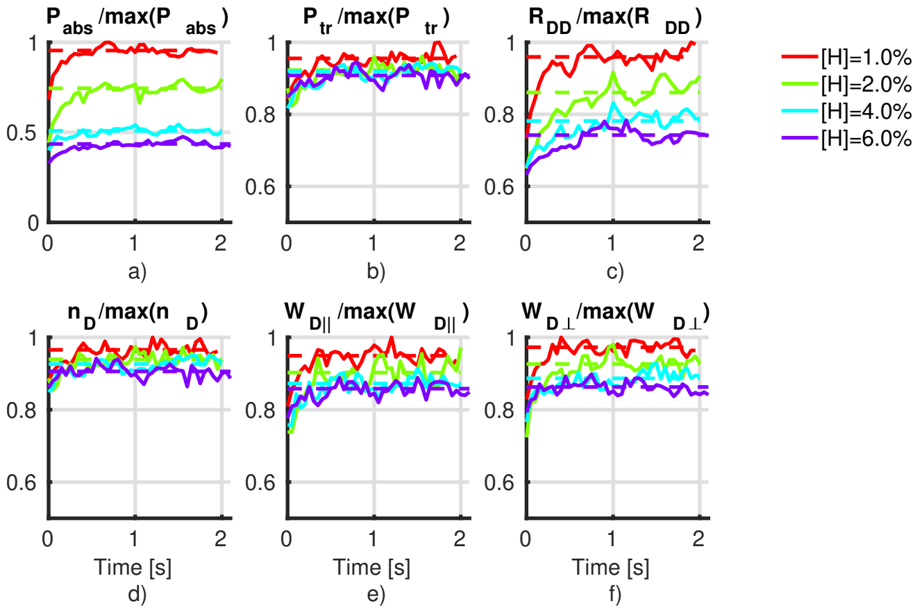
FIGURE 4.24: Évolution des quantités globales du plasma des modélisations auto-cohérentes EVE/SPOT pour différentes concentrations d'H (1%, 2%, 4%, 6%). a) Évolution de la puissance ICRH absorbée par le D rapide. b) Évolution de la puissance NBI et ICRH transférée au plasma. c) Évolution du taux de neutrons de la réaction D-D. d) Évolution de la densité de D rapide. e) Évolution du contenu énergétique parallèle du D rapide. f) Évolution du contenu énergétique perpendiculaire du D rapide.
