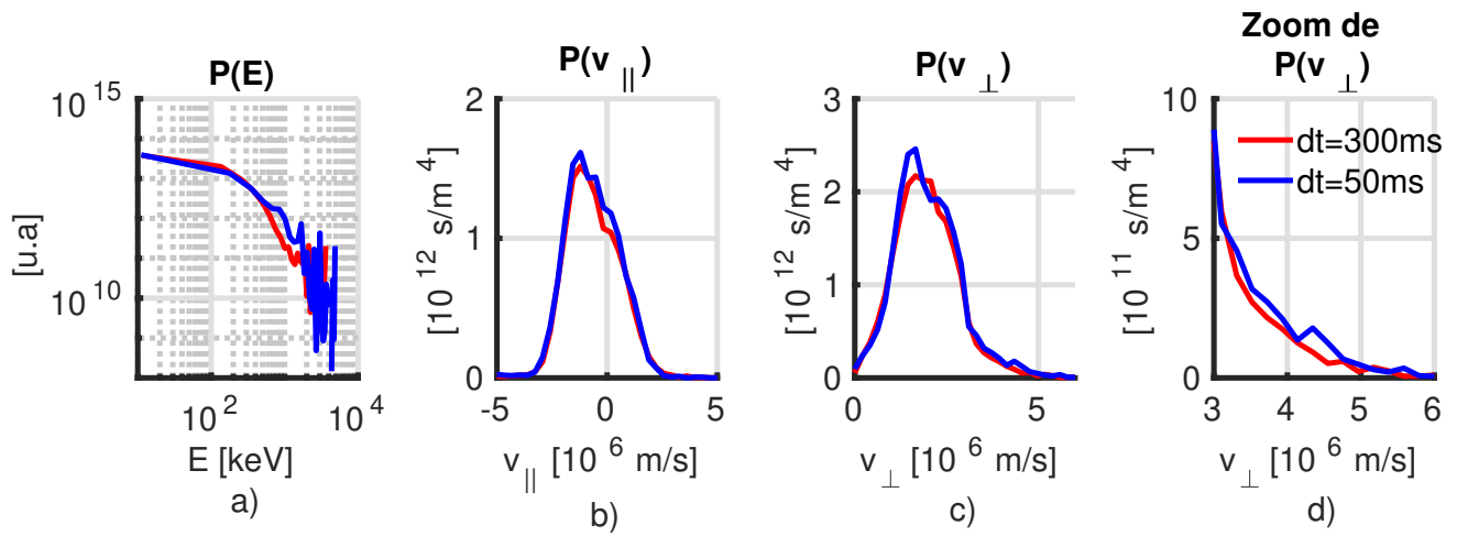
FIGURE 4.12: Comparaison de la distribution énergétique (a), de la distribution en vitesse parallèle (b) et perpendiculaire (c et d) du D rapide à \rho/\rho_0 = 0.1 entre deux simulations auto-cohérentes EVE/SPOT, une dont le temps d'évolution de la distribution dt entre chaque itération est de 50ms (en bleu) et une autre où dt vaut 300ms (en rouge).
