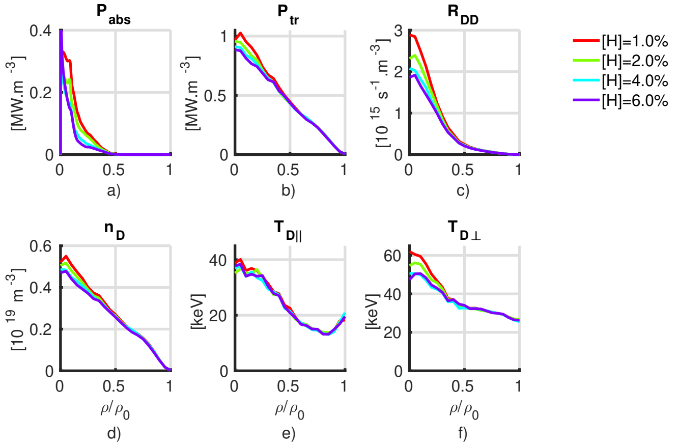
FIGURE 4.25: Comparaison des profils des modélisations auto-cohérentes EVE/SPOT pour différentes concentrations d'H (1%, 2%, 4%, 6%). a) Profils de la puissance ICRH absorbée par le D rapide b) Profils de la puissance transférée au plasma. c) Profils du taux de neutrons de la réaction D-D. d) Profils de la densité de D rapide. e) Profils de la température effective parallèle du D rapide. f) Profils de la température effective perpendiculaire du D rapide.
