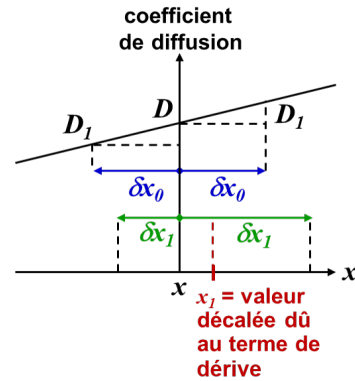
FIGURE 3.9: Représentation du calcul de l'opérateur Monte-Carlo pour l'interaction onde/particule
