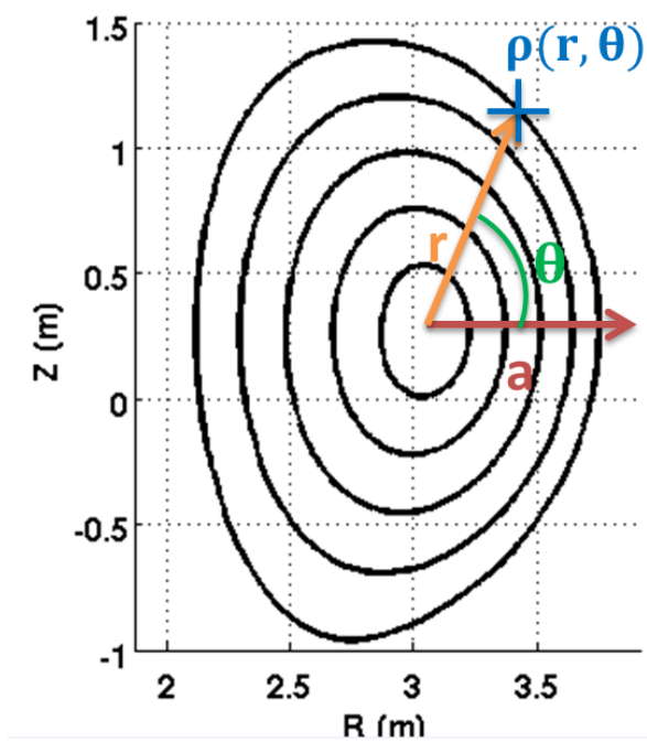
FIGURE 4.3: Schéma du changement de coordonnées entre le petit rayon plasma a et la coordonnée de flux toroïdal \rho . En noir sont représentées les surfaces de flux magnétique.
