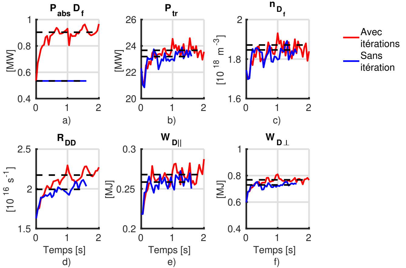
FIGURE 4.15: Comparaison de l'évolution temporelle des quantités globales du plasma entre la simulation auto-cohérente avec itérations entre EVE et SPOT (en rouge) et la simulation de SPOT sans itération avec EVE (en bleu). a) Évolution de la puissance ICRH absorbée par le D rapide. b) Évolution de la puissance transférée aux ions et électrons du plasma. c) Évolution de la densité du D rapide. d) Évolution du taux de neutrons de la réaction D-D e) Évolution du contenu énergétique dans la direction parallèle. f) Évolution du contenu énergétique dans la direction perpendiculaire.
