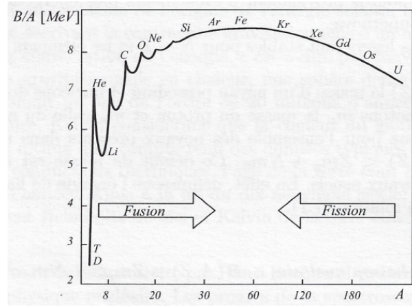
FIGURE 1.1: Energie de liaison par nucléon B(A, Z)/A [1]
