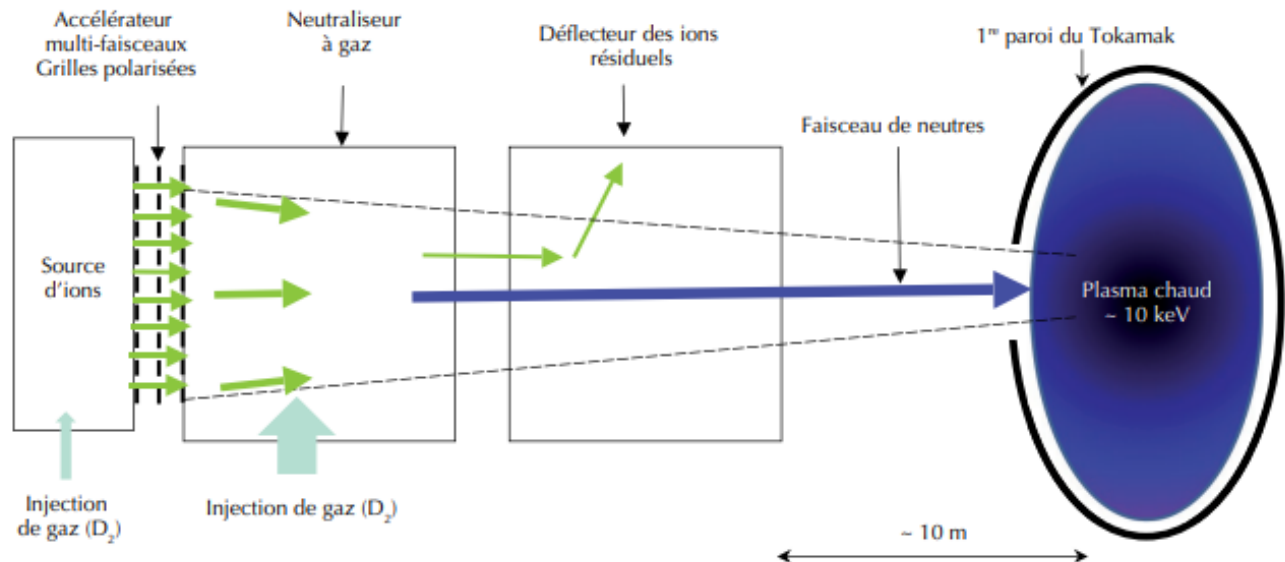
FIGURE 2.1: Principe d'une ligne d'injection de neutres. [7]
