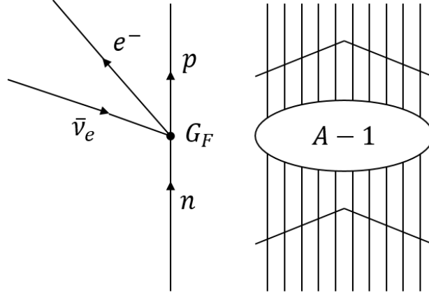
FIGURE 3.6 – Diagramme de Feynman d'une transition \beta^- dans le cadre de la théorie de Fermi et de l'approximation soudaine.
