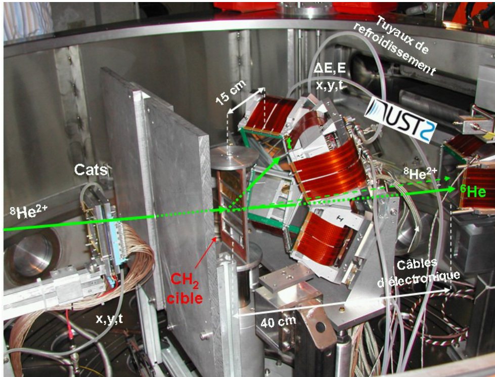
FIGURE 3 – Configuration du dispositif expérimental. Le plastique, couplé à un guide de lumière et une photodiode, a été rajouté par la suite devant et au centre du télescope à 40 cm de la cible. Un écran de protection a été placé entre la cible et le détecteur de faisceau Cats le plus proche.
