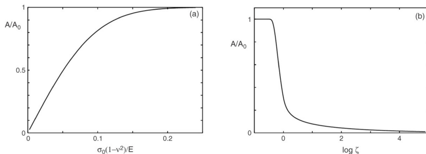
FIGURE 1.3 – Évolution de l’aire de contact relative obtenue par PERSSON (voir Persson (2006) pour les paramètres utilisés). La figure de gauche (a) présente l’évolution en fonction de la charge (au grossissement maximal) tandis que celle de droite (b) présente l’évolution en fonction du grossissement pour une charge donnée (fig. 10 de Persson (2006)).
