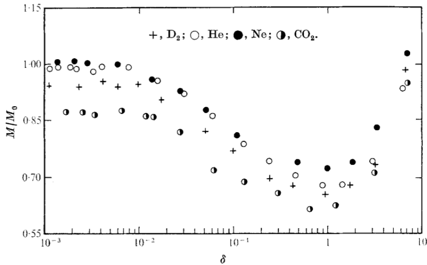
FIGURE 2.4 – Évolution de la conductance adimensionnelle en fonction du paramètre de raréfaction \delta \propto 1/\text{Kn} pour différents gaz dans une fente rectangulaire (d'après Porodnov et al. (1974) ).
