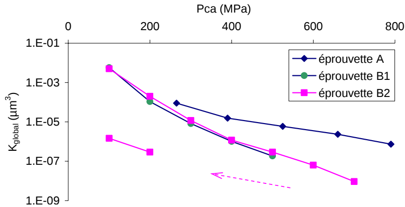
FIGURE 1.8 – Résultats expérimentaux donnant la transmissivité du contact en fonction de la pression d’assise pour trois éprouvettes (fig. 3.12 de Marie (2002)). La flèche indique des mesures faites lors de la décharge du contact.
