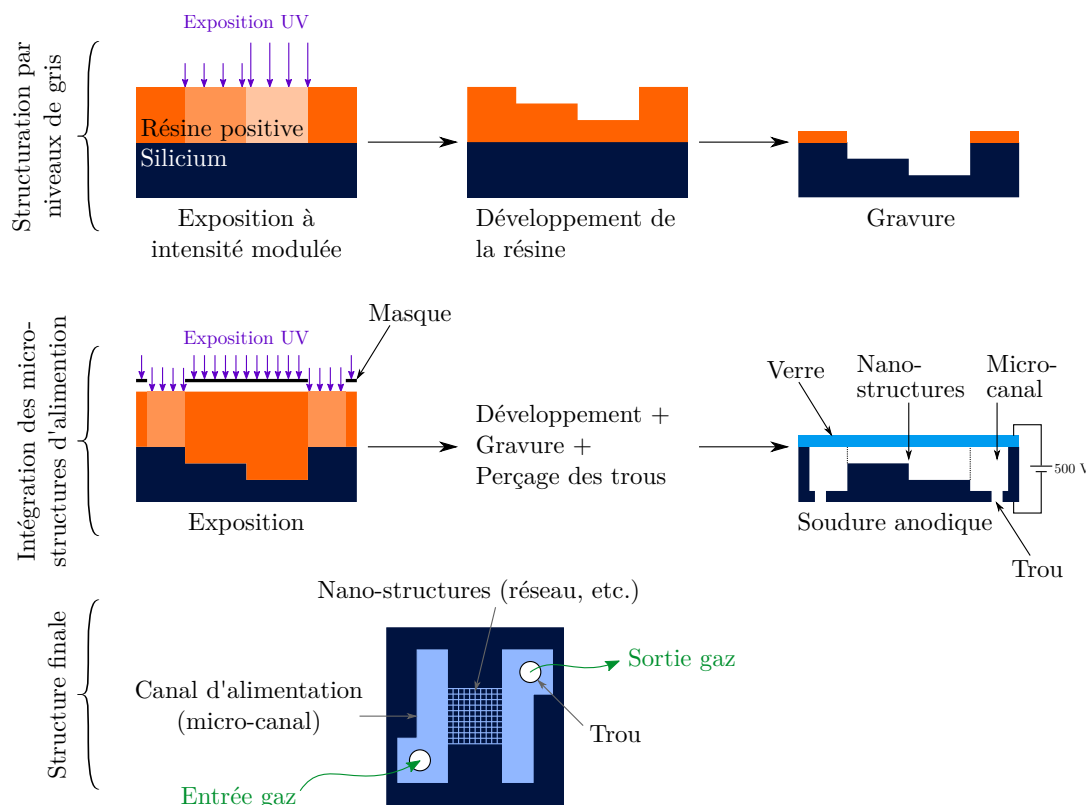
FIGURE 2.9 – Étapes de fabrication des puces nanofluidiques.
