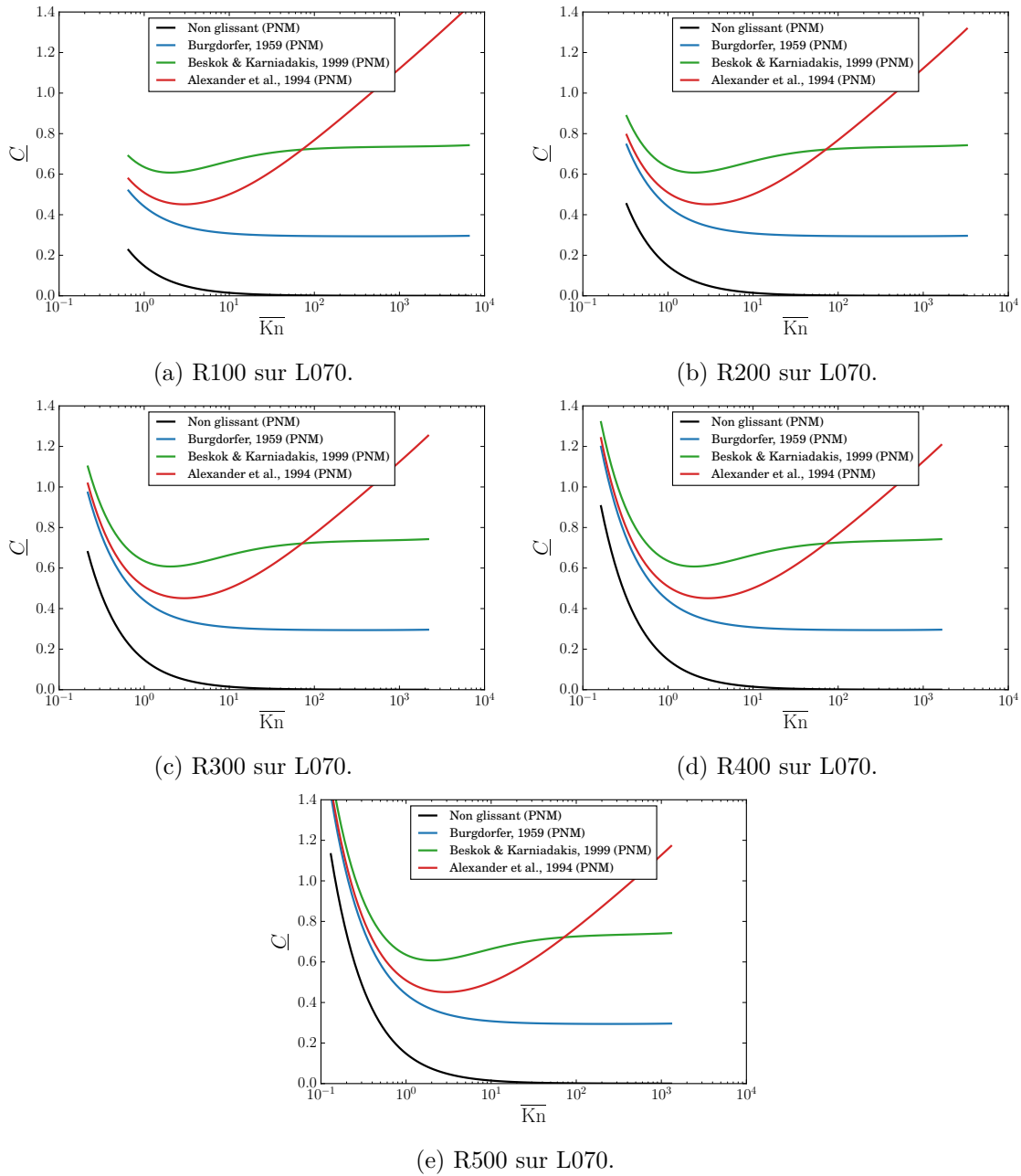
FIGURE B.3 – Réseaux homogènes du wafer L070.
