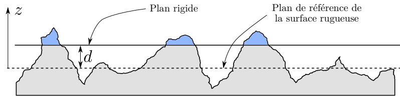
FIGURE 1.1 – Modélisation du contact selon Greenwood et Williamson (1966) . La charge est supportée par les aspérités d'altitude supérieure à d (en bleu).
