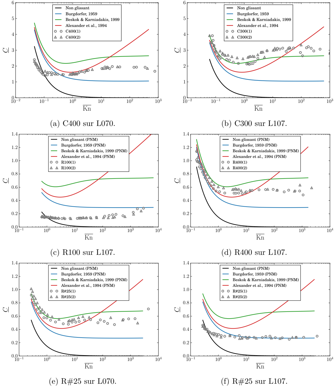
FIGURE 2.19 – Comparaison des résultats expérimentaux (points gris) aux différents modèles (traits pleins).
