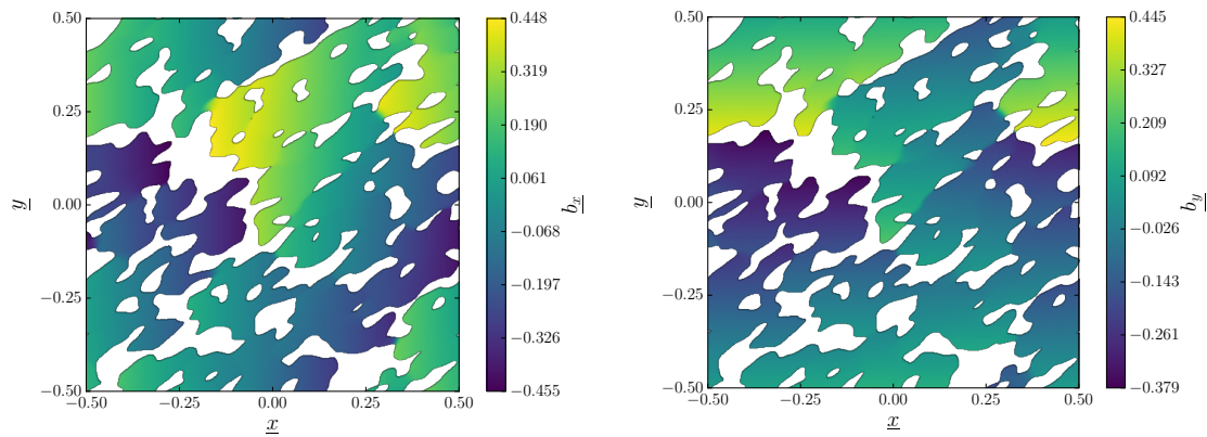
(a) \underline{b}_x = b_x/L_x pour \xi\overline{Kn} \approx 0,089 .
