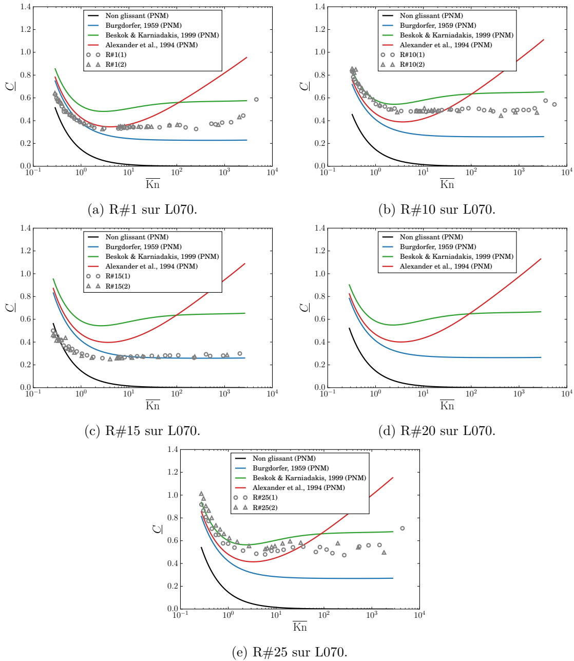
FIGURE B.5 – Réseaux hétérogènes du wafer L070.
