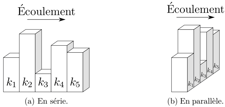
FIGURE 3.6 – Schématisation de l'arrangement de transmissivités.
