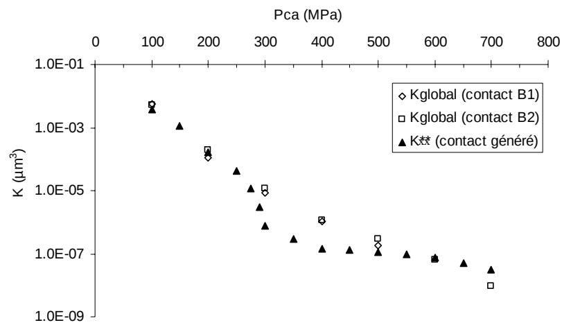
FIGURE 1.15 – Comparaison du débit de fuite calculé sur un contact complet avec le débit mesuré expérimentalement en fonction de la pression d'assise (fig. 4.48 de Marie (2002) ).
