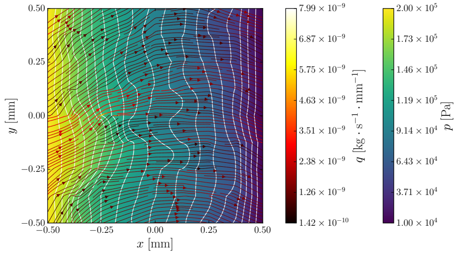
(a) Pression et lignes de courant.
