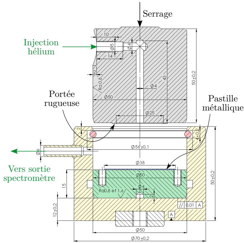
FIGURE 4.1 – Vue en coupe du dispositif expérimental de Tlili (2013) . Les constituants principaux sont : l'outil avec la portée rugueuse (gris) ; la pastille métallique (bleu) ; la pièce rectifiée (vert) ; le support (jaune) ; le joint torique (rouge).
