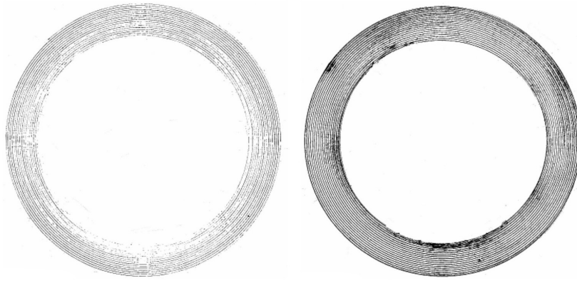
FIGURE 1.13 – Aire de contact (noire) mesurée à l’aide d’un film polymère de 1 \mu\text{m} d’épaisseur sur un joint en cuivre de 5 mm de largeur pour une pression d’assise de 12 MPa (à gauche) et 75 MPa (à droite) (fig. 6 de Nitta et Matsuzaki (2010) ).
