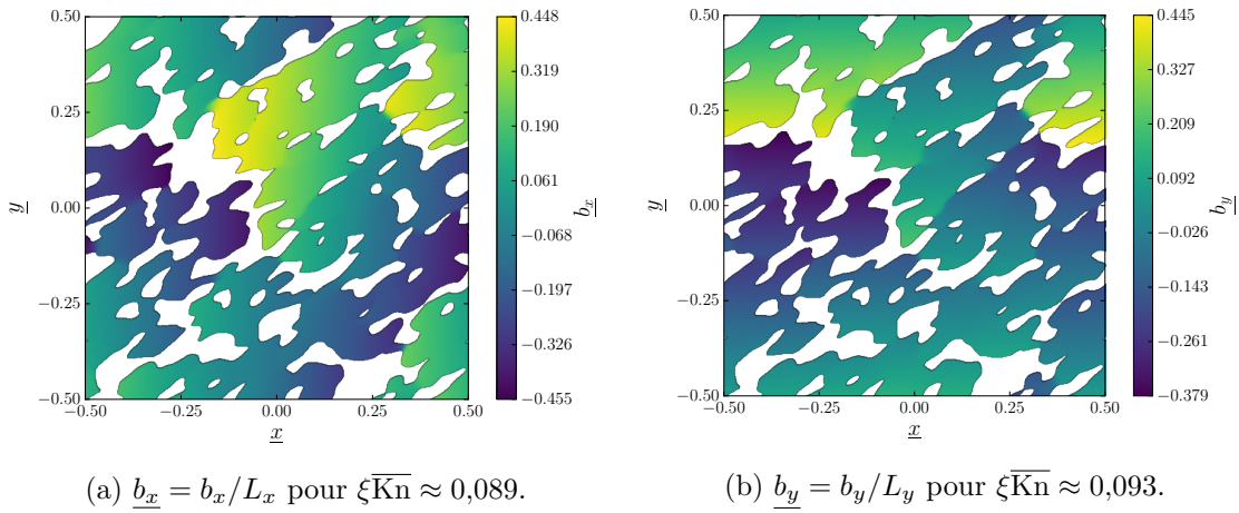
FIGURE 3.9 – Variables de fermeture adimensionnelles calculées pour le champ des ouvertures de la figure 3.3. Les longueurs de la surface sont rendues adimensionnelles comme \underline{x} = x/L_x et \underline{y} = y/L_y .
