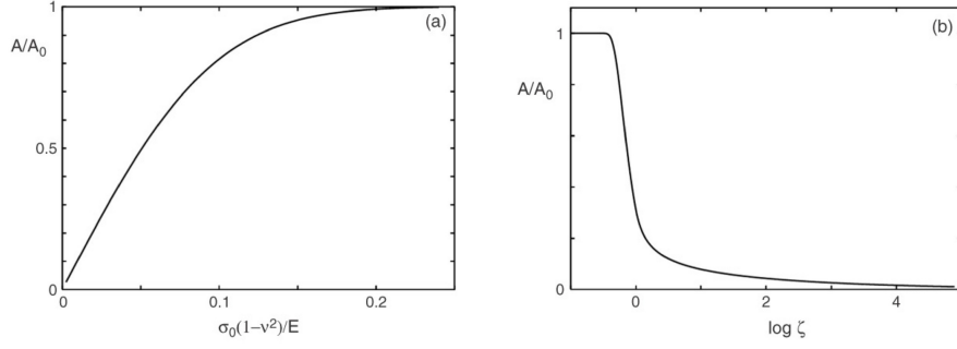
FIGURE 1.3 – Évolution de l'aire de contact relative obtenue par PERSSON (voir Persson (2006) ) pour les paramètres utilisés). La figure de gauche (a) présente l'évolution en fonction de la charge (au grossissement maximal) tandis que celle de droite (b) présente l'évolution en fonction du grossissement pour une charge donnée (fig. 10 de Persson (2006) ).
