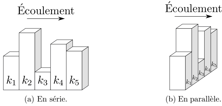
FIGURE 3.6 – Schématisation de l'arrangement de transmissivités.
