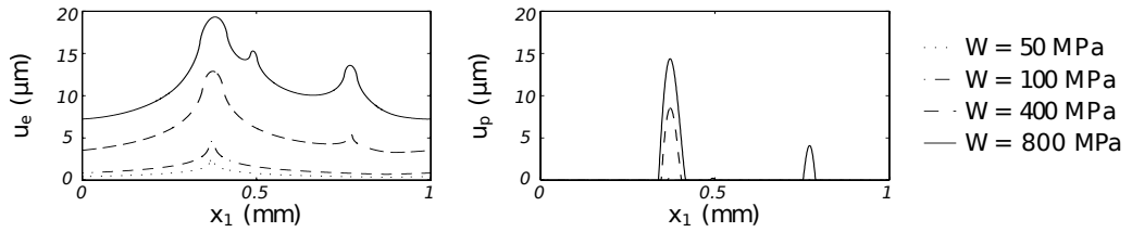
FIGURE 1.6 – Composante élastique (à gauche) et plastique (à droite) du déplacement de la surface pour différentes charges le long d'un contact (portion de la figure E.4 de Sahlin (2008)). Le déplacement plastique permanent augmente avec la charge.
