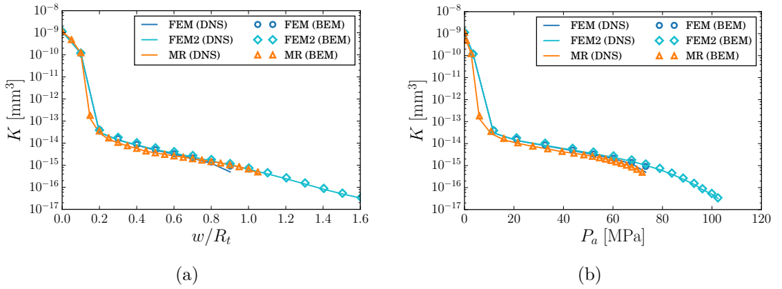
FIGURE 3.33 – Transmissivité apparente glissante en fonction de l'enfoncement adimensionnel ou de la pression d'assise. La légende indique d'abord le modèle de contact utilisé (FEM ou MR), puis entre parenthèses, la méthode pour le calcul d'écoulement (DNS ou BEM).
