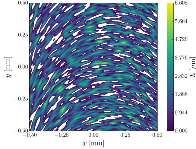
FIGURE 3.26 – Champ des ouvertures gaussien anisotrope, avec un taux de portance \varepsilon_\sigma = 17\% . Les zones blanches désignent des zones de contact.
