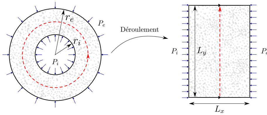
FIGURE 3 – Vue bidimensionnelle de la fracture sous forme annulaire (à gauche), et sa version « déroulée » selon le périmètre moyen (à droite).
