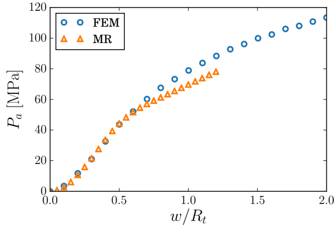
FIGURE 3.30 – Évolution de la pression d'assise en fonction de l'écrasement, obtenue par les éléments finis (FEM) et le modèle réduit (MR) pour la surface sans aspérités.
