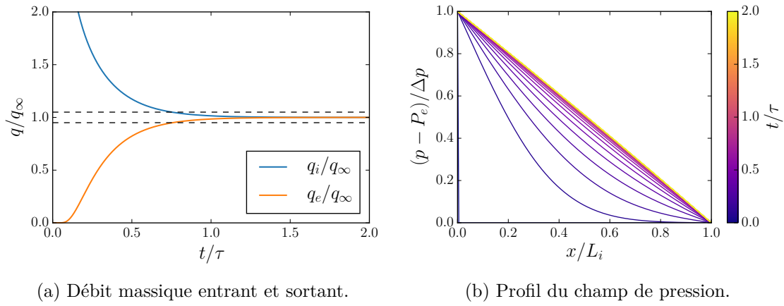
FIGURE 2.14 – Évolution temporelle des débits entrant et sortant d'un canal, ainsi que du champ de pression à un échelon en entrée. Le débit stationnaire est noté q_\infty , les débits entrant et sortant q_i et q_e respectivement. Les traits pointillés indiquent \pm 5\% de la valeur finale q_\infty .
