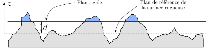
FIGURE 1.1 – Modélisation du contact selon Greenwood et Williamson (1966) . La charge est supportée par les aspérités d'altitude supérieure à d (en bleu).
