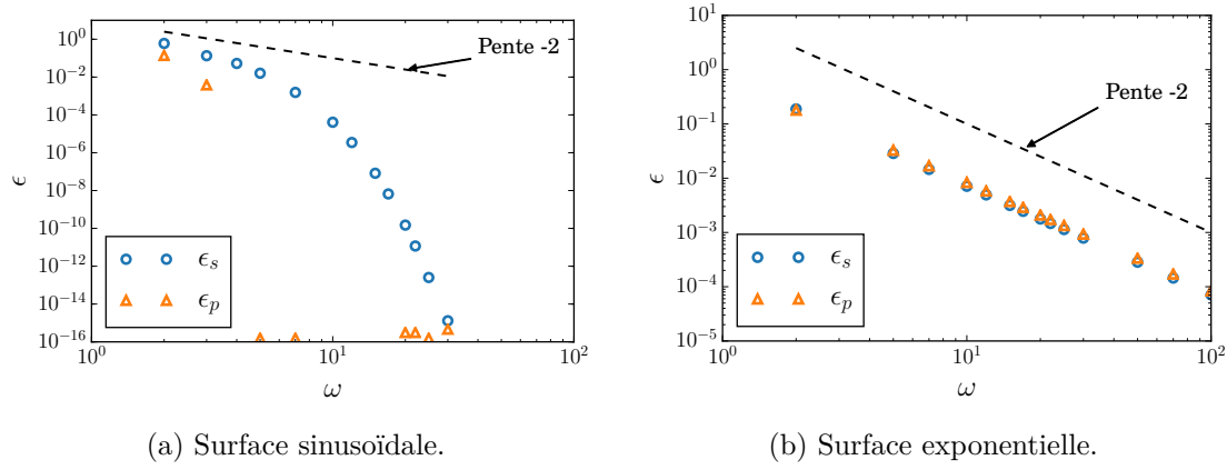
FIGURE 3.7 – Variation de l'erreur relative donnée par l'équation (3.126) entre les solutions analytique et numérique en fonction de la densité du maillage, \omega . La ligne en pointillés indique une loi puissance en \omega d'exposant -2 .
