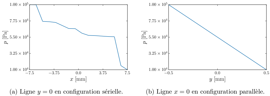
FIGURE 3.25 – Champ de pression le long de lignes particulières de la figure 3.24.
