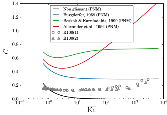
(c) R100 sur L107.
