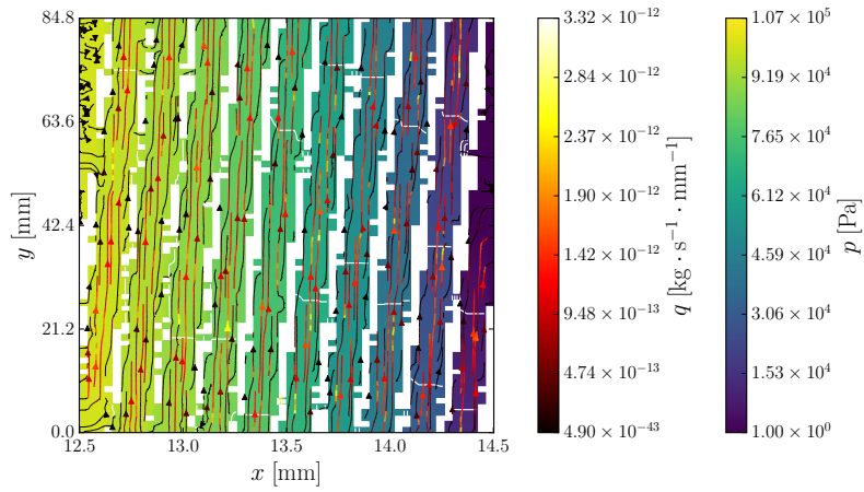
(a) BEM pour la surface MR – w/R_t = 0,5 .
