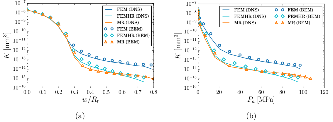
FIGURE 3.37 – Transmissivité apparente glissante en fonction de l'enfoncement adimensionnel ou de la pression d'assise. La légende indique d'abord le modèle de contact utilisé (FEM, FEMHR ou MR), puis entre parenthèses, la méthode pour le calcul d'écoulement (DNS ou BEM).
