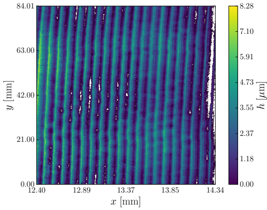
(c) Ouverture à P_a = 14 MPa (haute résolution).
