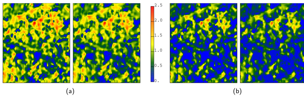
FIGURE 1.7 – Comparaison du champ des ouvertures entre un calcul par éléments finis (à gauche) et le modèle réduit (à droite) pour deux valeurs de déplacement imposé ( 0,89 \mu\text{m} en (a) et 1,35 \mu\text{m} en (b)). Les zones bleues sont les zones de contact (fig. 4.12 de Durand (2012)).
