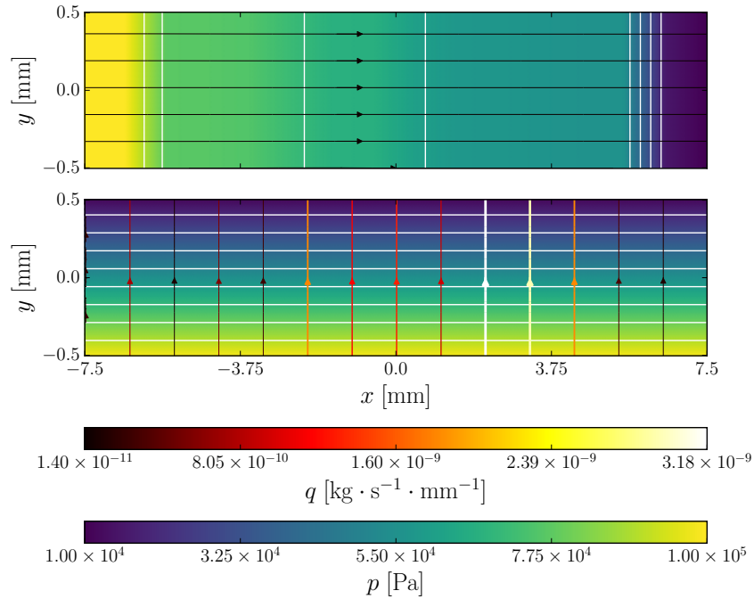
FIGURE 3.24 – Champs internes calculés par la méthode à deux échelles en configuration d'écoulement sérielle (haut) et parallèle (bas). Le champ de pression est présenté avec les couleurs allant du bleu au jaune, les lignes blanches correspondent aux isobares. Les lignes fléchées sont les lignes de courant du vecteur flux massique par unité de largeur, leur couleur indiquant la norme du vecteur.
