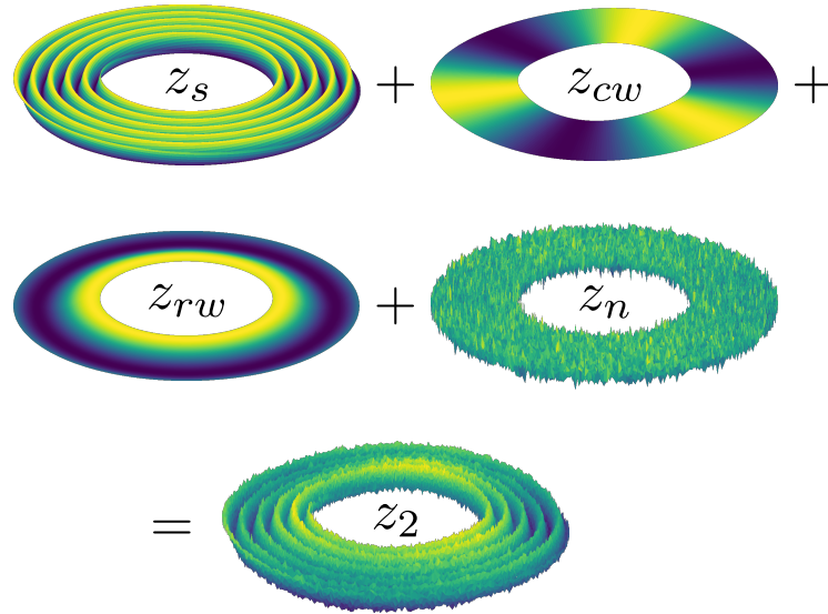
FIGURE 3.29 – Illustration schématique sous forme « non-déroulée » des différents modes composant une surface spiralée.
