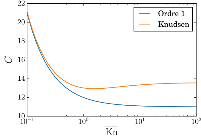
FIGURE 2.3 – Évolution de la conductance adimensionnelle en fonction du nombre de KNUDSEN pour le modèle de KNUDSEN (2.28) et pour le modèle de POISEUILLE glissant (2.29) (en prenant \xi = 16/3\pi\beta \approx 1,37 ).
