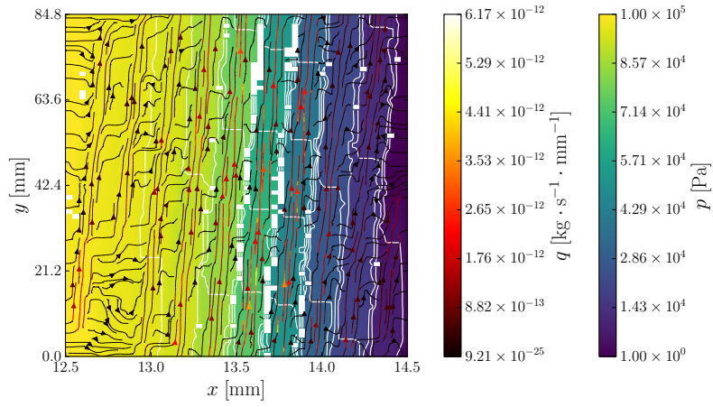
(b) BEM pour la surface FEMHR – w/R_t = 0,5 .
