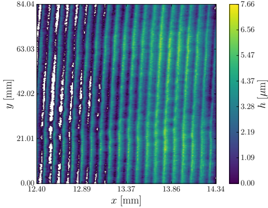
(e) Ouverture à P_a = 12 MPa (basse résolution).
