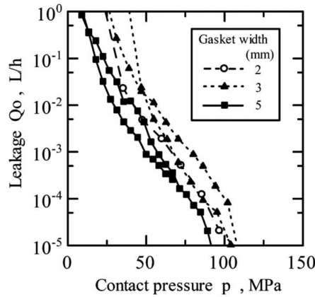
FIGURE 1.12 – Débits de fuite expérimentaux en fonction de la pression d'assise pour des joints en cuivre de différentes largeurs (fig. 4 de Nitta et Matsuzaki (2010) ).
