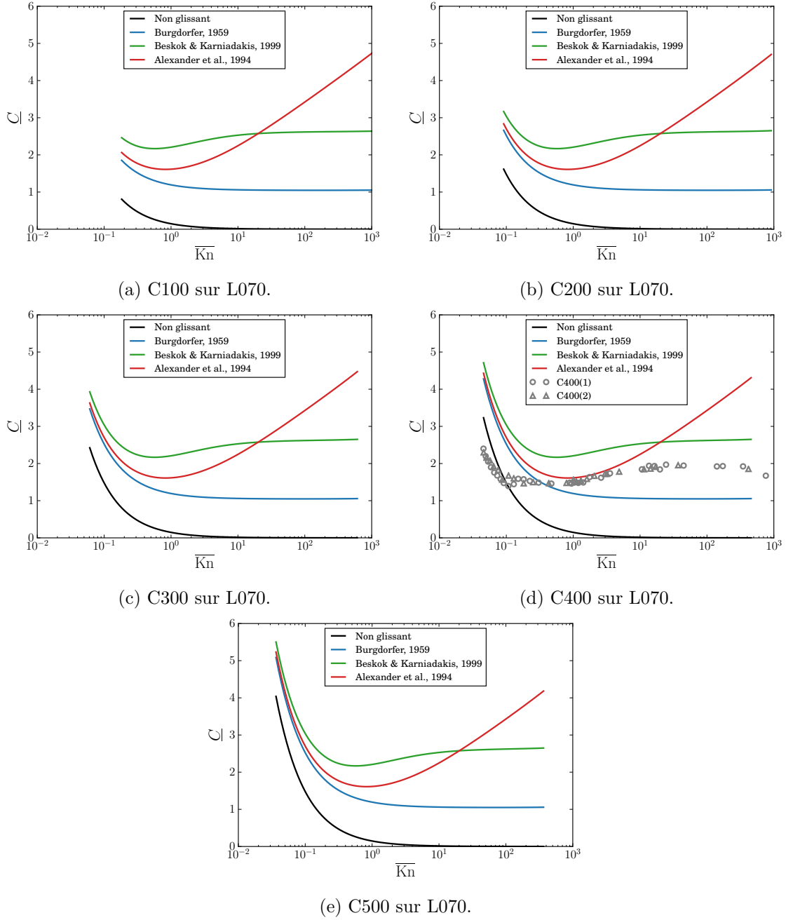
FIGURE B.1 – Canaux droits d'ouverture uniforme du wafer L070.
