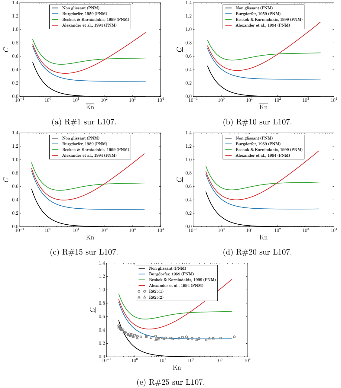
FIGURE B.6 – Réseaux hétérogènes du wafer L107.
