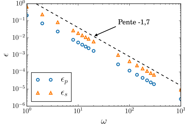
FIGURE 3.23 – Évolution des écarts relatifs des équations (3.183) entre les solutions analytiques et les solutions calculées par la méthode à deux échelles, en fonction de la densité du maillage \omega .
