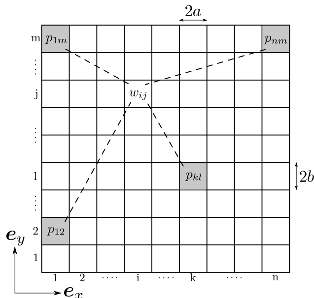
FIGURE 1.5 – Vue de dessus d’une grille de discrétisation du contact, avec quatre éléments en contact (c’est-à-dire ayant une pression de contact non-nulle; en gris).
