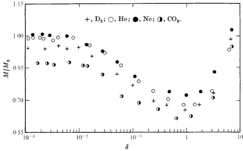
FIGURE 2.4 – Évolution de la conductance adimensionnelle en fonction du paramètre de raréfaction \delta \propto 1/\text{Kn} pour différents gaz dans une fente rectangulaire (d'après Porodnov et al. (1974) ).
