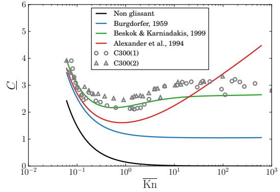
(b) C300 sur L107.
