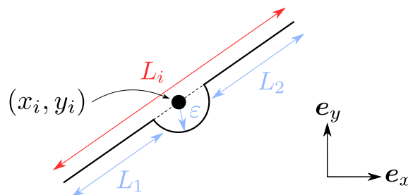
FIGURE E.1 – Paramétrisation de l'élément i (de longueur L_i ) pour le calcul de G_{ii} et H_{ii} .
