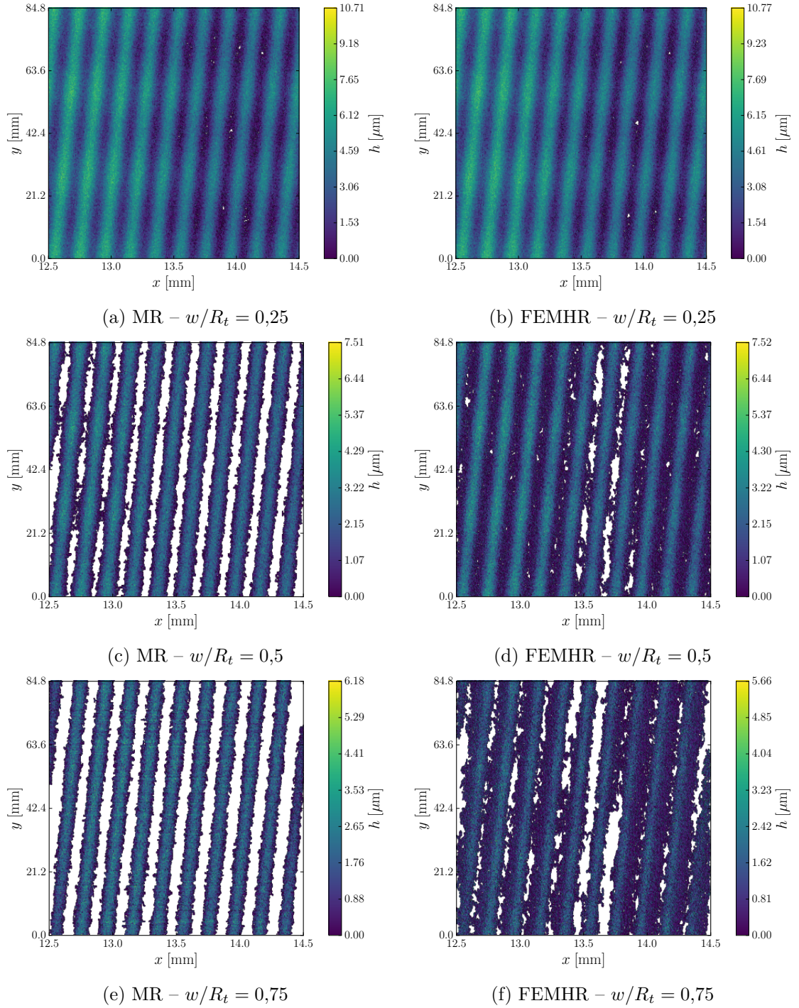
FIGURE 3.35 – Évolution du champ des ouvertures en fonction de l'enfoncement adimensionnel selon le modèle numérique de contact utilisé (FEMHR ou MR) pour le profil avec aspérités. Les zones blanches sont des zones de contact.
