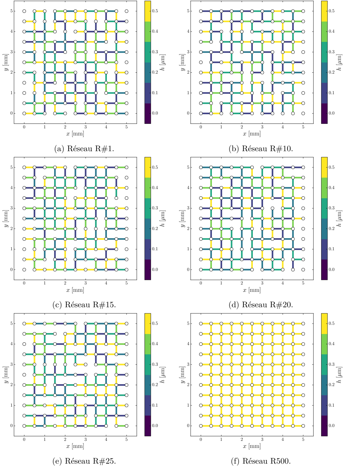
FIGURE A.1 – Géométrie des réseaux hétérogènes et d'un réseau homogène. La couleur donne la profondeur gravée des liens.
