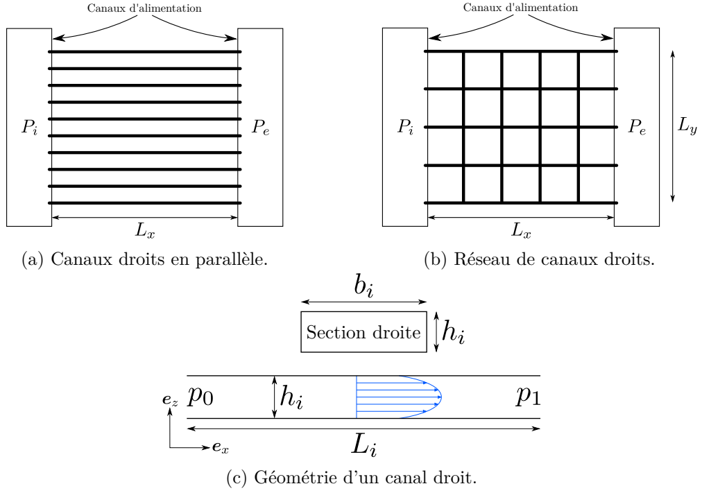
FIGURE 2.7 – Schéma des deux types de puces réalisées. On représente également les canaux d'alimentation aux extrémités des puces, permettant l'apport et l'extraction du gaz.
