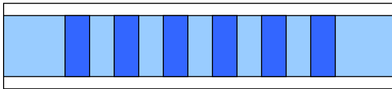
Figure 1.16 – Réseau de Bragg dans une fibre optique (les couleurs différentes correspondent aux indices différents)
