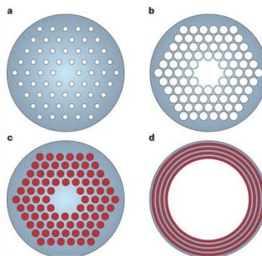
Figure 1.3 – Types différents des fibres à cristaux photoniques : a – fibre monomode à cœur silice ; b – fibre à cœur creux ; c – fibre remplie de liquide, d – fibre creuse multicouche [7 Knight]
