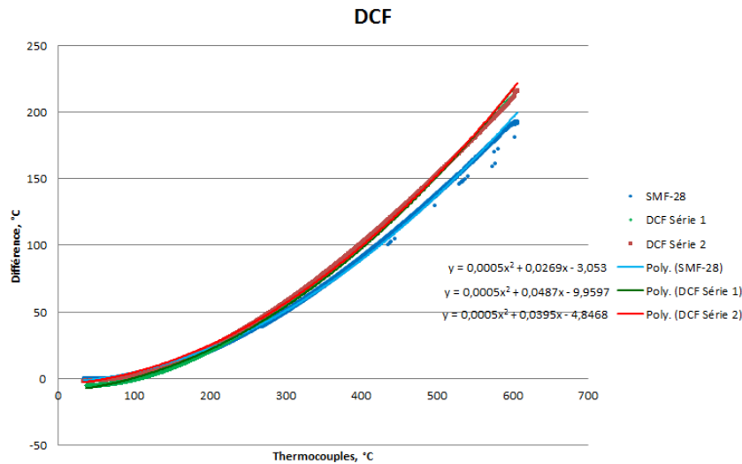
Figure 3.8 – Différence entre la température mesurée par les thermocouples et par l’OBR pour la fibre DCF (rouge et vert) et pour la fibre SMF-28 (bleu)
