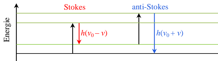
Figure 1.22 – Explication du processus de formation des raies Stokes et anti-Stokes de la diffusion Raman
