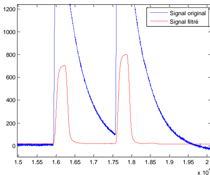
Figure 1-21 : Résultat du filtre trapézoïdal configuré pour diminuer le risque d'empilements.
