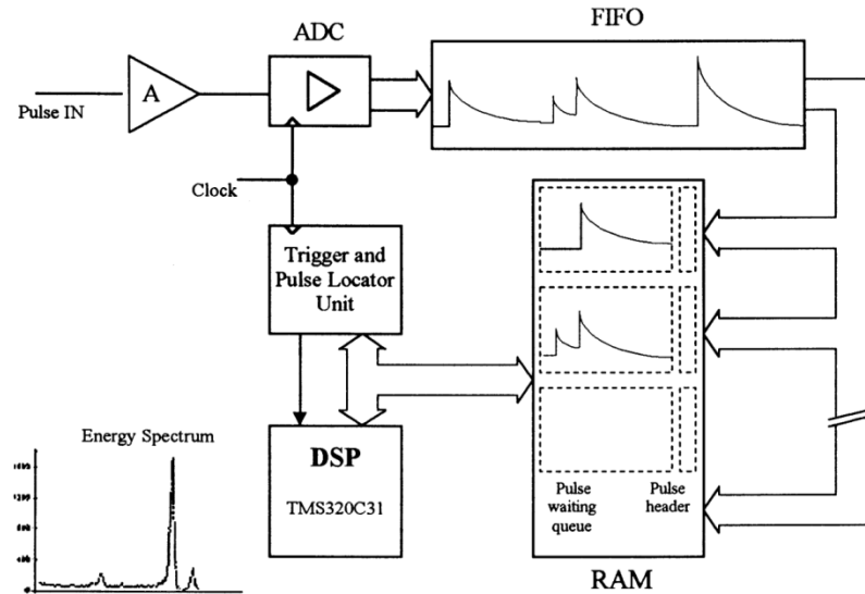
Figure 1-28 : Gestion de la mémoire du DPP de Cardoso.
