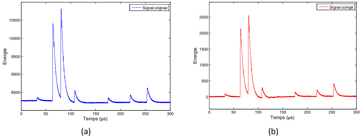
Figure 1-19: Illustration d'une correction de ligne de base avec (a) une fraction du signal original et (b) le signal corrigé
