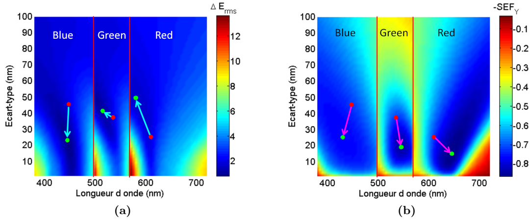
FIGURE 3.45 – Variation (a) de l'erreur colorimétrique, (b) du SEF en fonction de la longueur d'onde pic des filtres colorés et de leur largeur.
