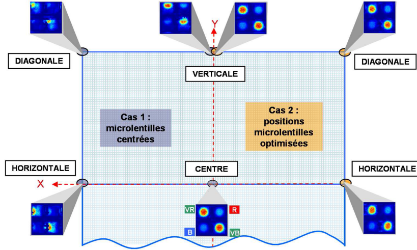
FIGURE 3.21 – Simulation des pixels sur l'axe optique et hors d'axe, pour des microlentilles uniformément réparties (cas 1), ou pour des microlentilles dont le placement est optimisé suivant la position dans le champ de l'image
