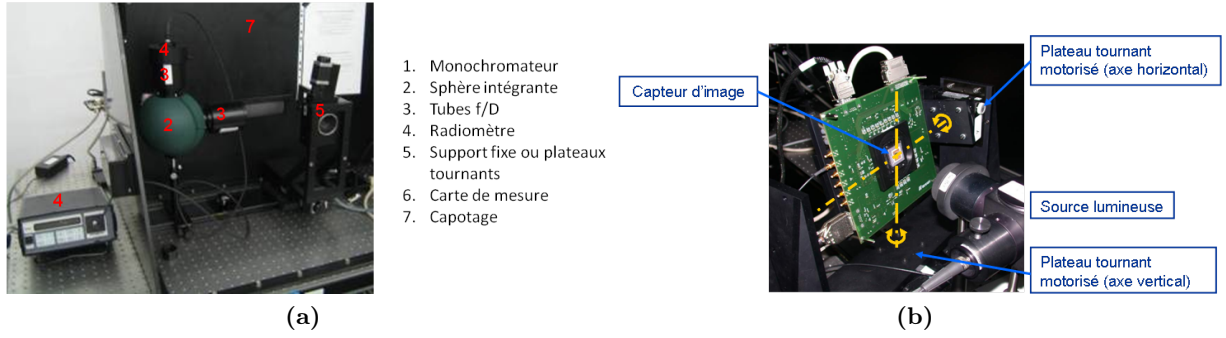
FIGURE 3.39 – Banc de caractérisation du rendement quantique avec un angle de rayon principal arbitraire (a), capteur monté sur les platines de rotation afin d'émuler l'angle de rayon principal (b)
