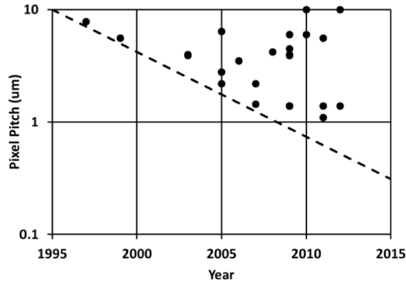
FIGURE 3.3 – Évolution de la taille des pixels aux cours des deux dernières décennies sur la base des articles publié, la courbe en pointillé montre la tendance de réduction du pas[2].
