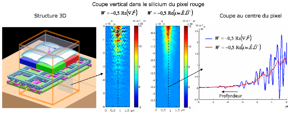
FIGURE 3.34 – Comparaison de la génération optique calculée suivant les formules 3.11 et 3.13
