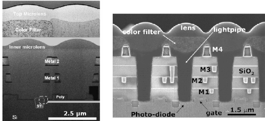
FIGURE 3.28 – Coupe d'un pixel de 2,5\mu\text{m} avec une lentille interne, source Sony [25] (à gauche), et d'un pixel de 2,2\mu\text{m} avec guide d'onde, source IBM [26] (à droite)
