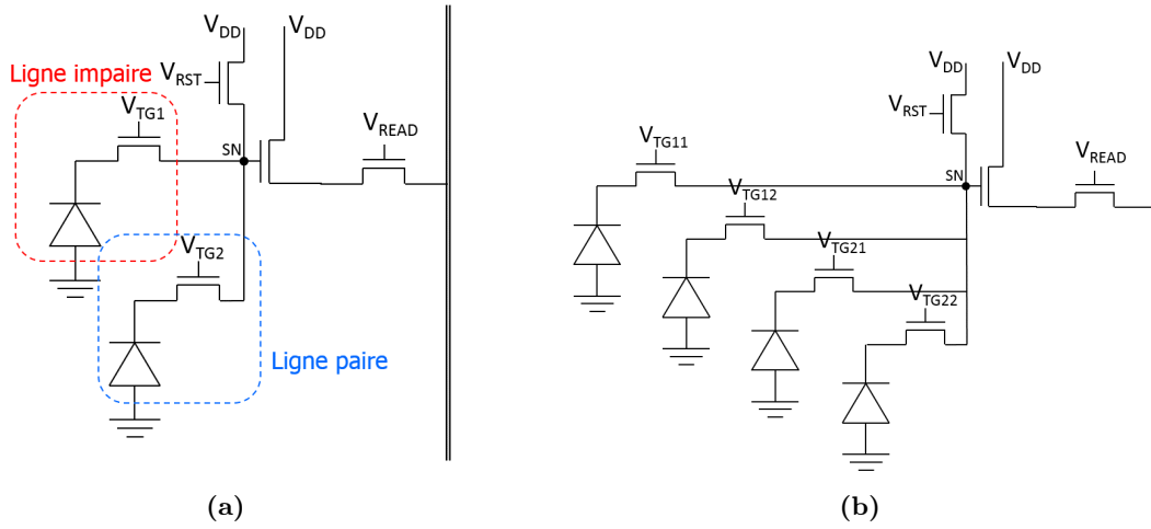
FIGURE 3.9 – Architecture de pixel à partage de transistors : (a) 2T5 soit cinq transistors pour deux pixels, (b) 1T75 soit sept transistors pour quatre pixels
