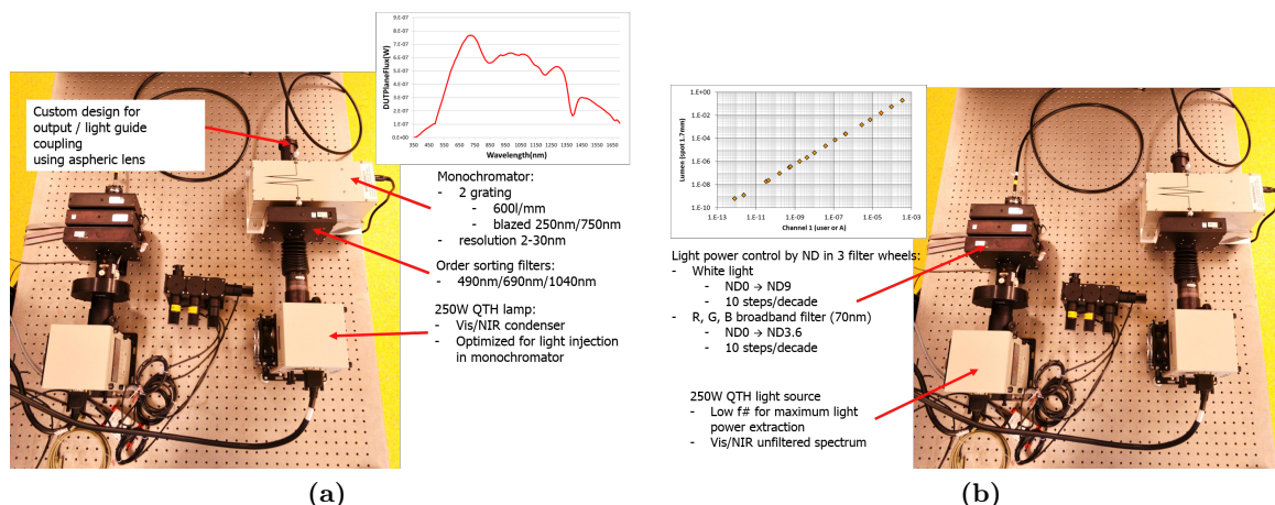
FIGURE 4.2 – Sources monochromatique (a), blanche (b) et LED au milieu
