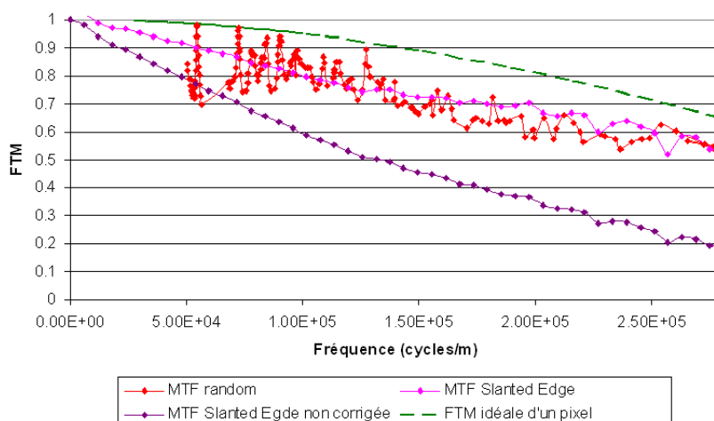
FIGURE 3.14 – Comparaison entre les mesures par bord de plage (brute en violet, corrigée de l'optique en magenta) et la mesure par mire pseudo-aléatoire (rouge)
