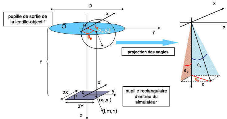
FIGURE 3.18 – Source utilisée pour le tracé de rayon sous Zemax permettant la simulation en éclairment diffus ou collimaté
