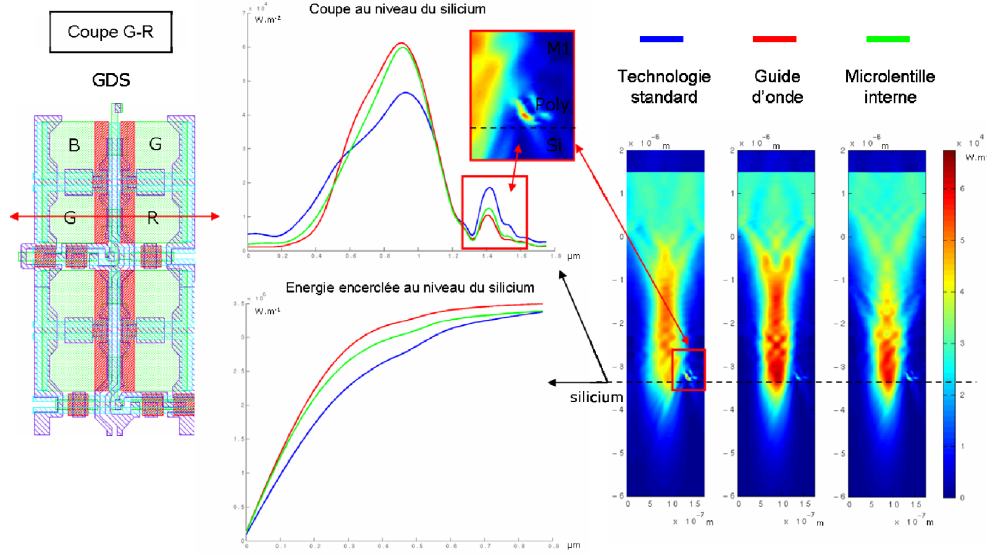
FIGURE 3.29 – Comparaison des solutions standard, avec guide d'onde et avec microlentille interne dans le cas d'un pixel fortement asymétrique
