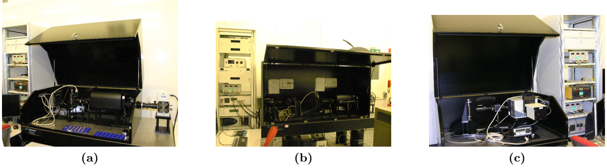
FIGURE 3.12 – Bancs optiques développés pour la caractérisation des images (a) en lumière blanche (b) sous incidence oblique (c) du rendement quantique.
