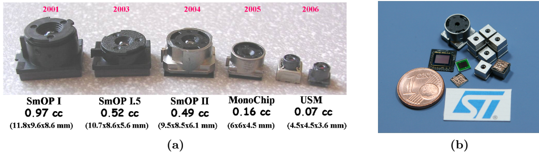
FIGURE 3.4 – Évolution de la taille des caméras miniatures : (a) pour un capteur de définition VGA (0.3Mpixel) entre 2000 et 2006, (b) pour un capteur 2Mpixels entre les générations de pixel 3\mu m et 1,75\mu m , source STMicroelectronics.
