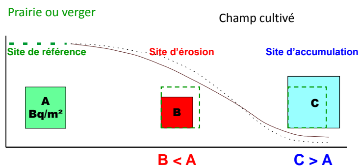
Figure 6 (Adapté de Bonté). Principe de la méthode des inventaires de ^{137}\text{Cs} pour calculer l'érosion des sols. Elle consiste à comparer l'inventaire en Bq/m 2 mesuré dans les champs cultivés (sites B et C) avec celui d'un site de référence (site A; n'ayant subi ni érosion ni accumulation).
