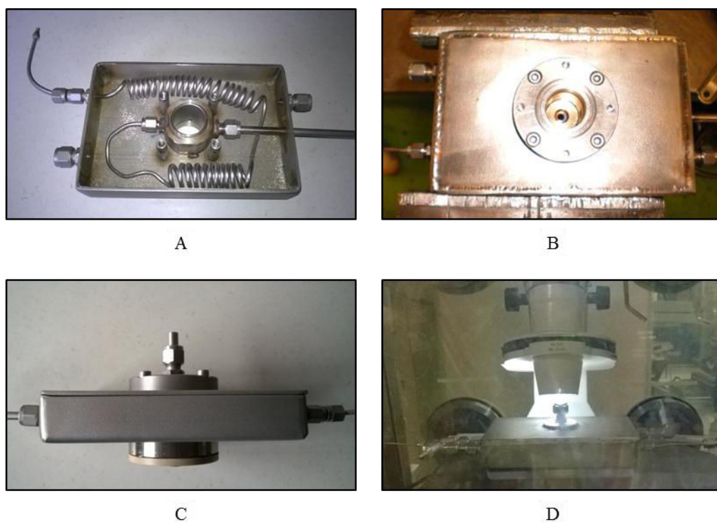
Figure 2.5 – Cellule de dissolution alimentée en continu et thermostatée : intérieur de la double-enveloppe (A), puits de réaction (B), vue d'ensemble de la cellule (C), et cellule sur le microscope (D)
