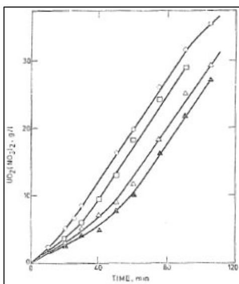
Figure 1.24 – Influence de la concentration de nitrite sur les cinétiques de dissolution : 0,05 molal NaNO_2 ( \square ), 0,01 molal NaNO_2 ( \blacksquare ), 0,001 molal NaNO_2 ( \triangle ), sans NaNO_2 ( \blacktriangle ) [SHA-69-01]
