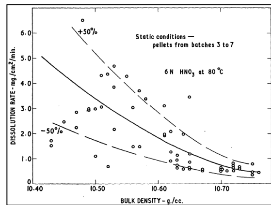
Figure 1.28 – Effet de la densité sur les vitesses de dissolution [TAY-62-01]
