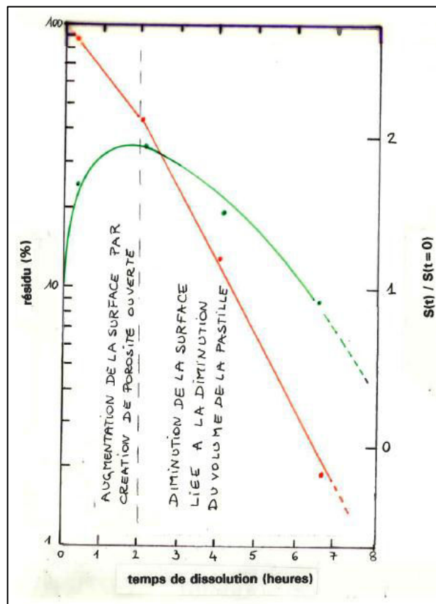
Figure 1.34 – Évolution de la surface spécifique au cours du temps (courbe verte) et comparaison avec le pourcentage dissout (courbe rouge) [PIL-92-01]
