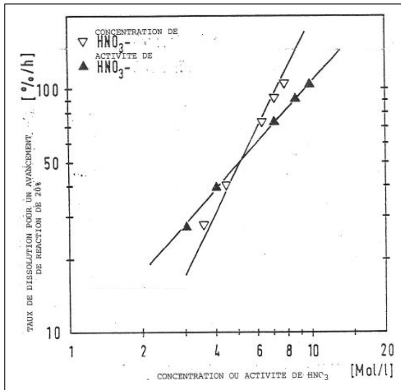
Figure 1.25 – Comparaison de l'évolution des vitesses de dissolution en fonction de la concentration d'acide nitrique (▽) et de son activité (▲) à 70 °C [HER-84-01]
