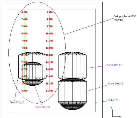
Figure 39 : Représentation de la modélisation VISIPLAN des cuves
