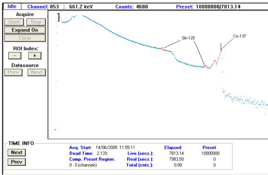
Figure 37: Spectre obtenu en champ ouvert avec un détecteur CdZnTe de volume sensible 20 mm 3
