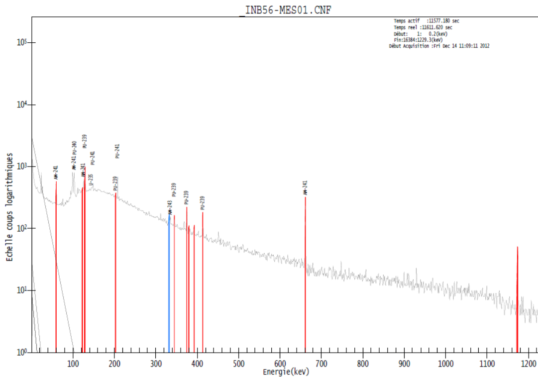
Figure 55 : Configuration de mesure par spectrométrie gamma et spectre gamma
