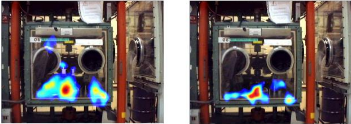
Figure 40 : Image d'une boîte à gants contenant une presse, à gauche image de caméra gamma équipée d'un sténopé, à droite image d'une caméra gamma équipée de masque codé
