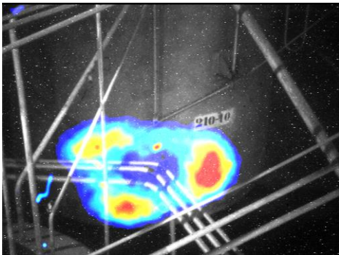
Figure 38 : Image gamma de la cuve 210-10
