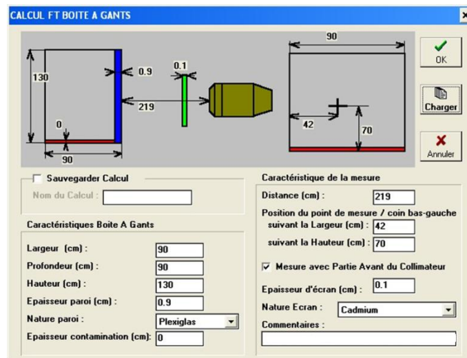
Figure 14 : Interface utilisateur du progiciel Ensemble de Mesure de Boites A Gants (EMBAG) pour le calcul de fonctions de transfert FT(E)
