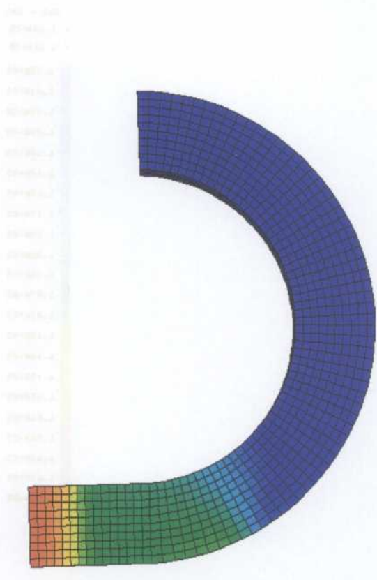
COUDE CHIMIE AVEC GLISSIERMENT 3D PRESSION (PA) - T(S) = 2.00000E-04
