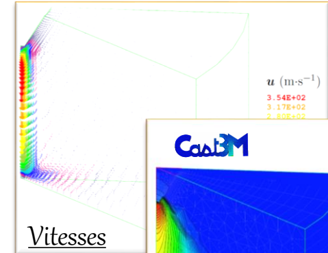
Soudage à l'arc TIG
