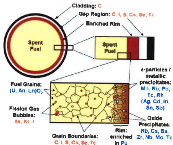
Figure 1 : Schéma de la microstructure d'un combustible utilisé représentant la distribution des actinides et des produits de fission [2].
