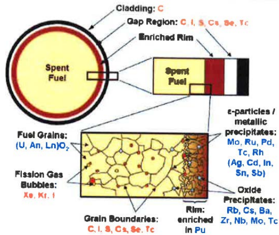
Figure 1 : Schéma de la microstructure d'un combustible usé représentant la distribution des actinides et des produits de fission [2].
