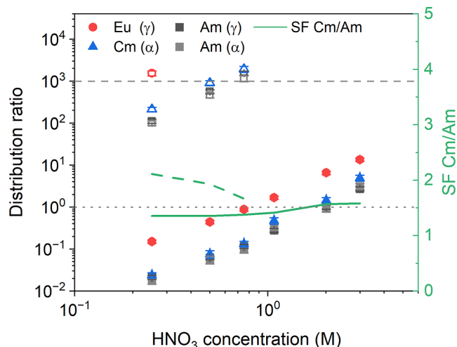
Figure 5. Influence of \text{HNO}_3 on iPDdDGA extraction. Aq: 10^{-3} mol·L ^{-1} Ln(III) + 3 kBq/mL ^{152}\text{Eu} , ^{241}\text{Am} , and ^{244}\text{Cm} radiotracers in x mol·L ^{-1} \text{HNO}_3 . Org: 0.1 mol·L ^{-1} (open symbols, dashed line) or 0.005 mol·L ^{-1} (closed symbols, full line) iPDdDGA dissolved in 10% _{\text{vol}} 1-octanol in n -dodecane, 2X pre-equilibrated with x mol·L ^{-1} \text{HNO}_3 . A/O: 1, 1900 rpm, T : 20 °C, shaking time: 15 min.
