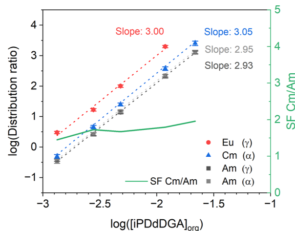
Figure 6. Slope analysis of iPdDdDGA extraction. Aq: 10^{-3} mol·L -1 Ln + 3 kBq/mL 152 Eu, 241 Am, and 244 Cm radiotracers in 3 mol·L -1 HNO 3 . Org: x mol·L -1 iPdDdDGA dissolved in 10% v/v 1-octanol in n -dodecane, 2× pre-equilibrated with 3 mol·L -1 HNO 3 . A/O: 1, 1900 rpm, T : 20 °C, shaking time: 15 min.
