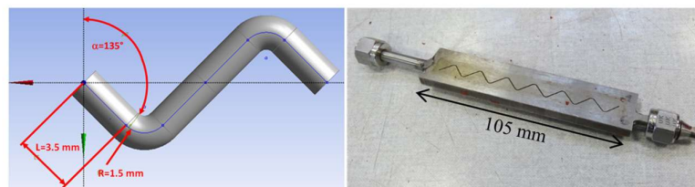
Figure 1 : Vue CAO du canal zigzag (à gauche) et photographie d'une maquette FA (à droite).
