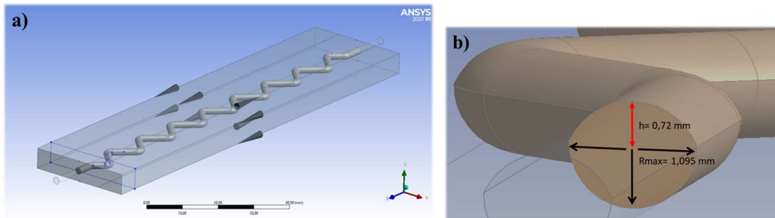
Figure 4 : Géométrie de calcul ; vue complète (à gauche) et zoom section de passage (à droite).
