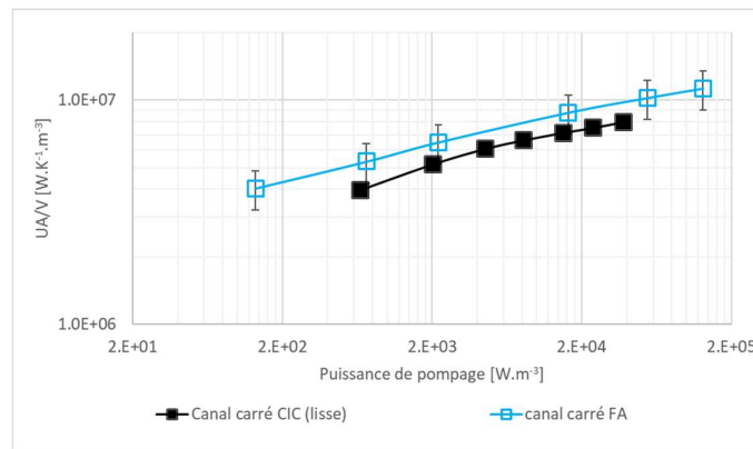
Figure 2 : Facteur d'intensification vs. puissance de pompage selon les deux procédés de fabrication.
