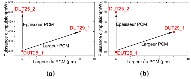
FIGURE 2. Puissance requise pour différentes largeurs et épaisseurs de commutateurs PCM : (a) pour l'amorphisation ; (b) pour la cristallisation.
