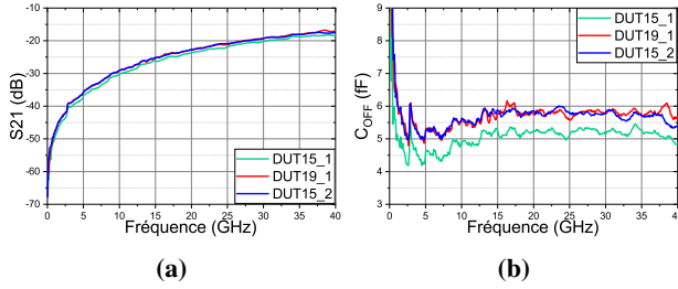
FIGURE 4. Performances RF du GeTe amorphe : (a) isolation ; (b) Capacité.
