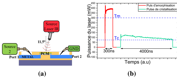
FIGURE 1. (a) Montage expérimental pour l'excitation optique ; (b) Exemple d'impulsions laser utilisées.
