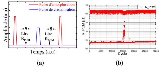
FIGURE 5. (a) Schéma de la synchronisation de la mesure du cyclage ; (b) Cycles de commutation.
