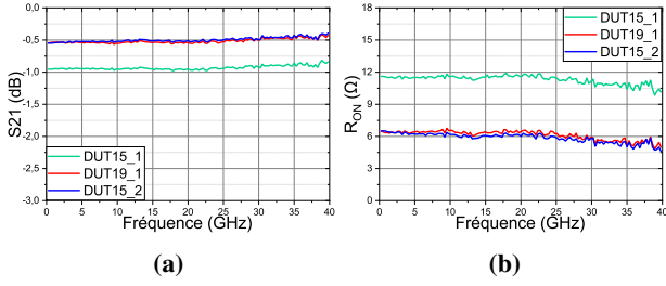
FIGURE 3. Performances RF du GeTe cristallin : (a) Perte d'insertion ; (b) Résistance.
