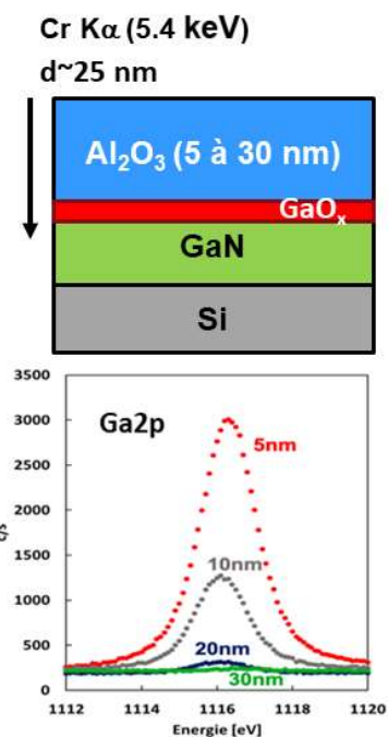
Figure 1. Schéma de l'empilement représentatif du HEMT et spectres Ga 2p 3/2 mesurés en source Cr K \alpha en fonction de l'épaisseur d'Al 2 O 3 .
