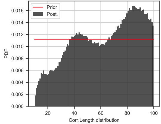
(d) Posterior corr.length distribution for v_{SW}
