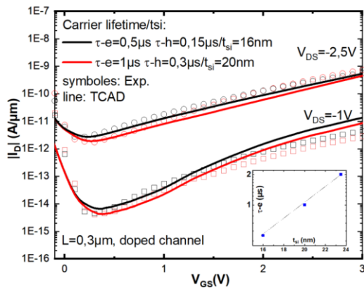
Fig. 10 : TCAD vs. EXP. I_D - V_{GS} for V_{DS}=-2.5V and V_{DS}=-1V .
