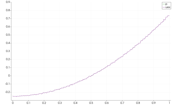
(d) Horizontal section on the random triangle mesh
