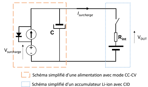
Figure 8 : schéma de test tel qu'indiqué dans les normes
