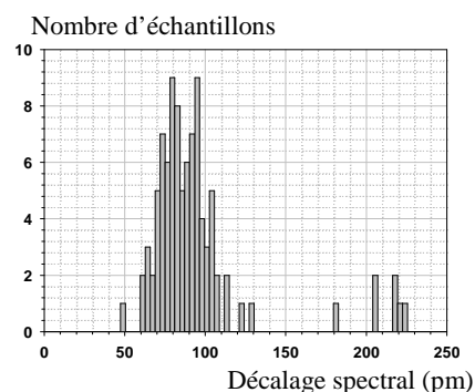
Fig. 4c : Distribution de la déformation moyenne d'une section de ligne de contact relevée pour une centaine de trains commerciaux
