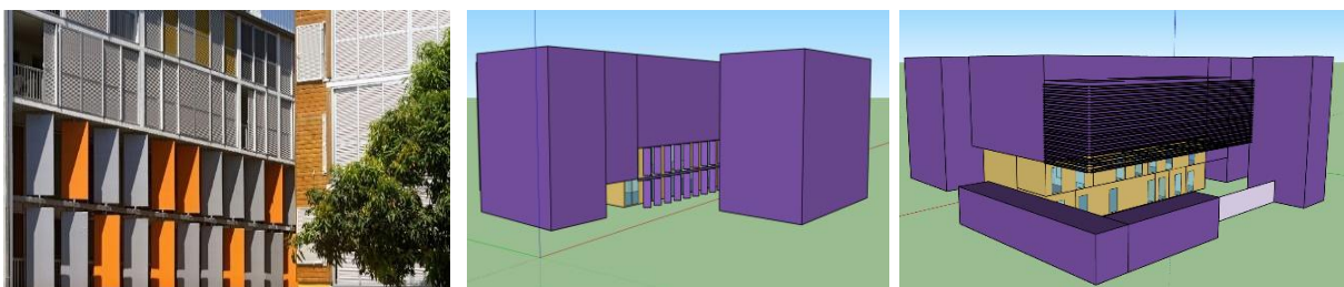
Figure 3 – Photographie et axonométries du bâtiment Ilet du Centre
