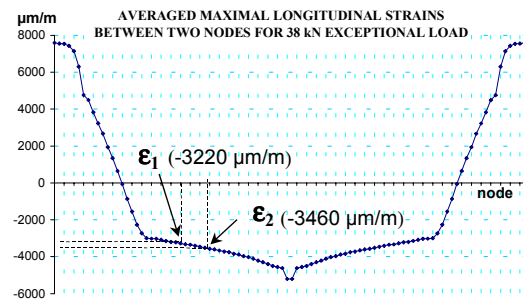
Fig. 12: SAMCEF® longitudinal strains modeling
