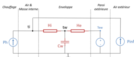
Fig. 5 : Modèle RC utilisé pour la calibration.
