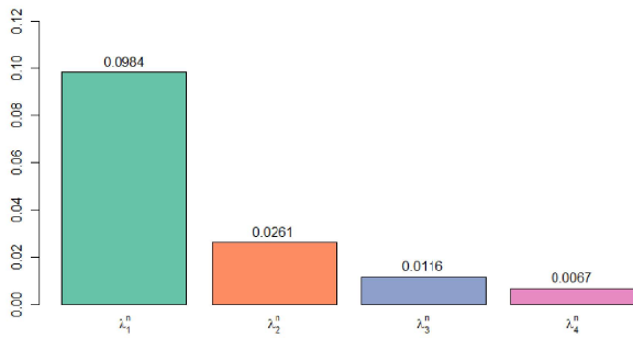
Eigenvalues
