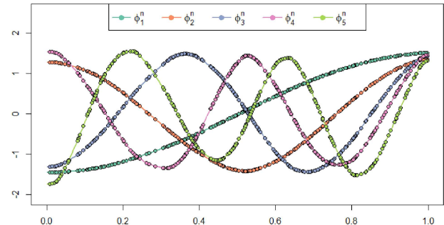
Eigenfunctions
