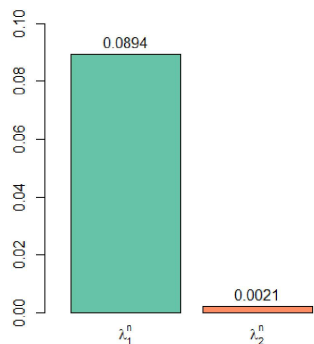
Eigenvalues
