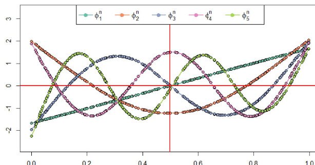
Eigenfunctions
