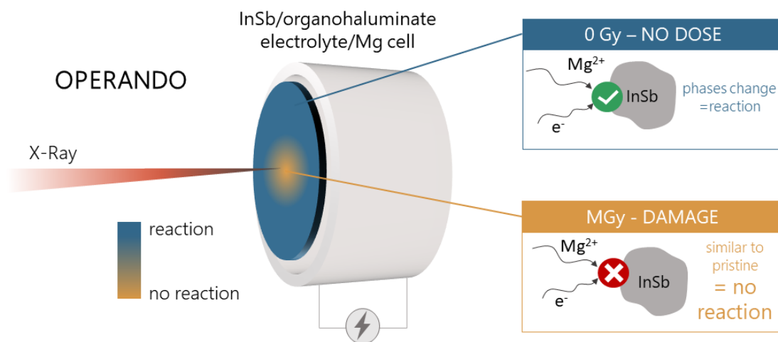
Figure 1 : Schéma représentant l'effet de faisceau observé operando sur une cellule InSb/électrolyte organohaluminat/Mg. Alors que les transformations de phase sont présentes dans toute l'électrode lors de la magnésiation, les changements de phase sont presque totalement annihilés sur la zone sondée par le faisceau.
