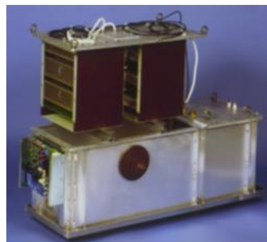
Figure 7 : commutateur 25 kV 2 kA ouvert
