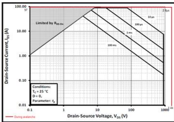
Figure 14 : courant d'avalanche d'un MOSFET SiC
