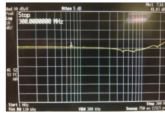
Figure 5 : comportement fréquentiel de la sonde réalisée
