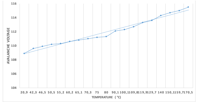
Figure 12 : tension d'écrêtage en fonction de la température
