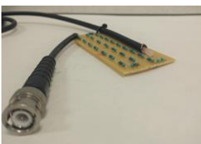
Figure 4 : sonde 5 kohm sortie 50 ohms
