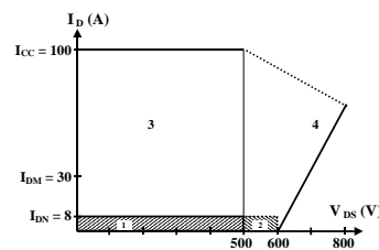
Figure 1: Aire de sécurité de l’IRF840
