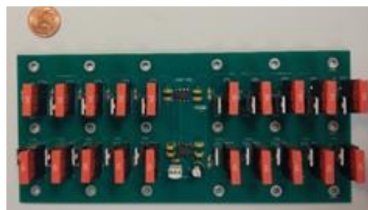
Figure 9 : Carte 2 kA constituée de 20 MOSFET
