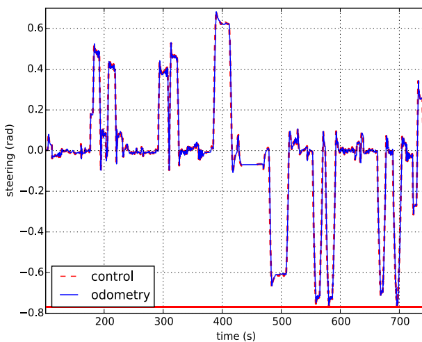
Fig. 18. Front steering angle.
