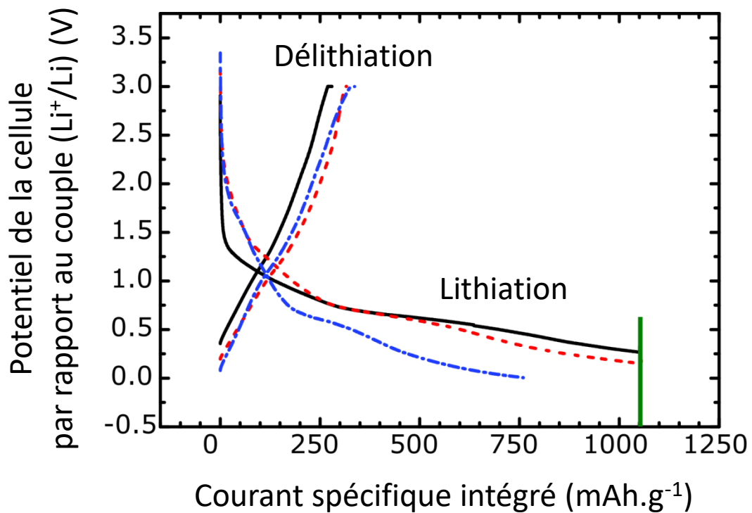
Figure 4 - Premier cycle de charge-décharge (cyclage galvanostatique) réalisé à courant constant entre 0 et 3 V pour l'échantillon de référence (trait plein noir) et deux échantillons irradiés à des doses croissantes : 92 kGy, (tirets rouge), et 202 kGy, (points-tirets bleu). La ligne verticale verte correspond au temps limite de l'expérience (60 heures). Figure issue de [14] et reproduite avec l'autorisation de la Royal Society of Chemistry.
