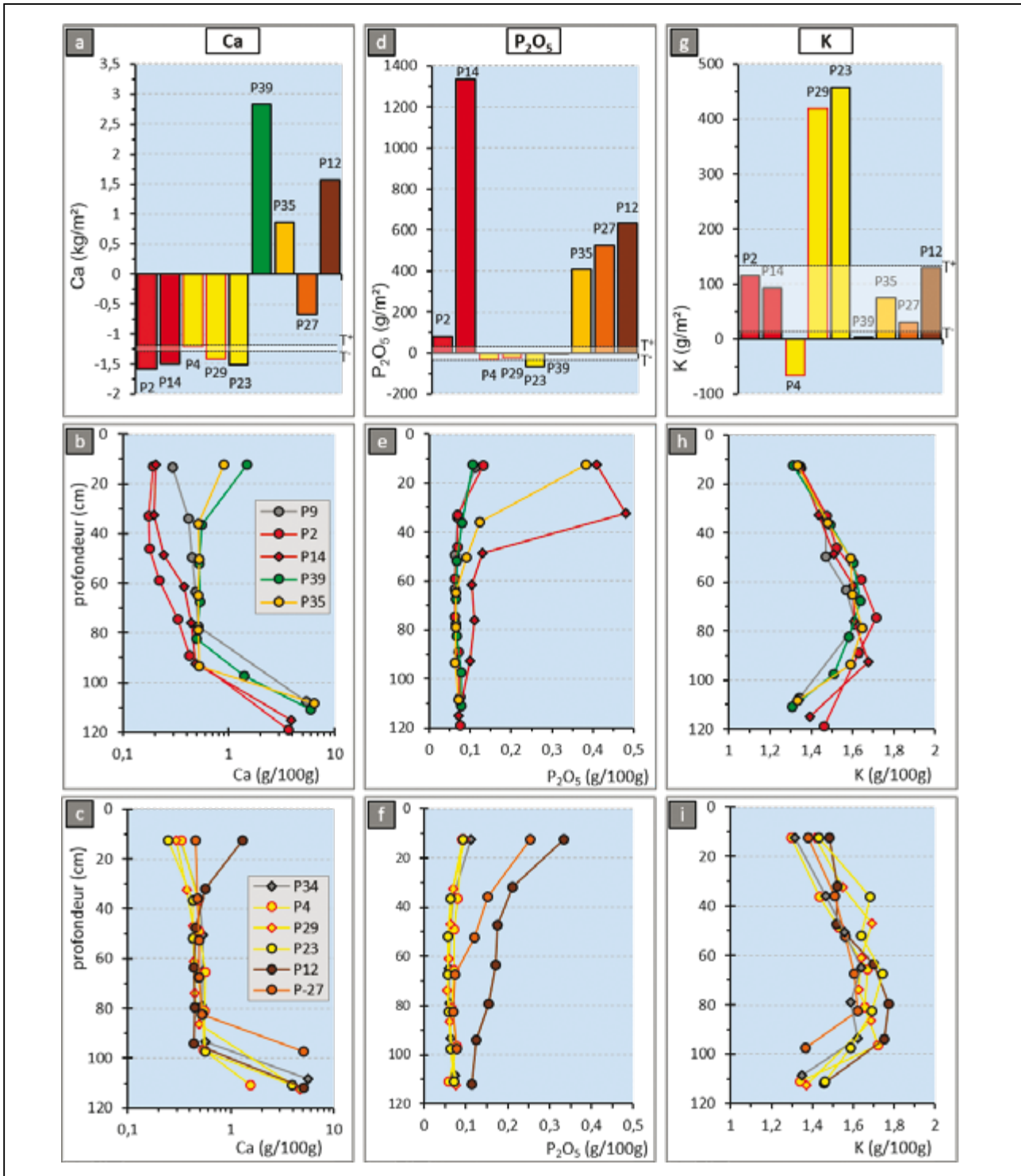
Figure 5 - Bilans géochimiques de Ca (a), P 2 O 5 (d) et K (g) dans les horizons de surface, et profils des concentrations en Ca (b,c), P 2 O 5 (e,f) et K (h,i) dans les horizons profonds. P9 : témoin ; P2 : sulfate d'ammonium ; P14 : phosphate di-ammonium ; P35 : scories ; P39 : carbonate de calcium ; P34 : témoin ; P4 : nitrate de sodium ; P29 : sylvinite ; P23 : chlorure de potassium ; P12 : fumier ; P27 : superphosphate. Figure 5 - Geochemical budgets for Ca (a), P 2 O 5 (d) and K (g) in surface horizons, and concentrations profiles of Ca (b,c), P 2 O 5 (e,f) and K (h,i) in soil depth. P9: reference; P2: ammonium sulphate; P14: ammonium phosphate; P35: basic slag; P39: calcium carbonate; P34: reference; P4: sodium nitrate; P29: sylvinite; P23: potassium chloride; P12: manure; P27: superphosphate.
