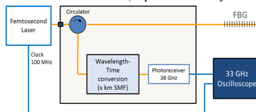
Fig. 3 : Spectromètre dynamique basé sur la dispersion et un système d'acquisition ultrarapide.
