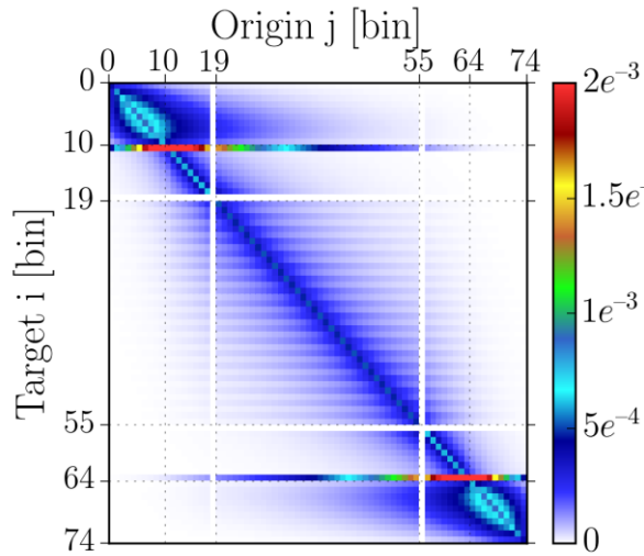
Figure 9: « prompt-to-delayed » fission matrix
