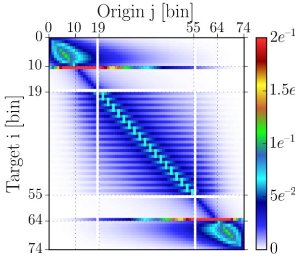
Figure 6: « prompt-to-prompt » fission matrix
