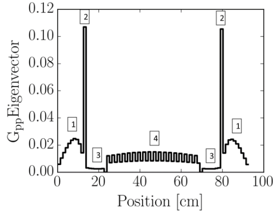
Figure 8: « prompt-to-prompt » fission matrix eigenvector
