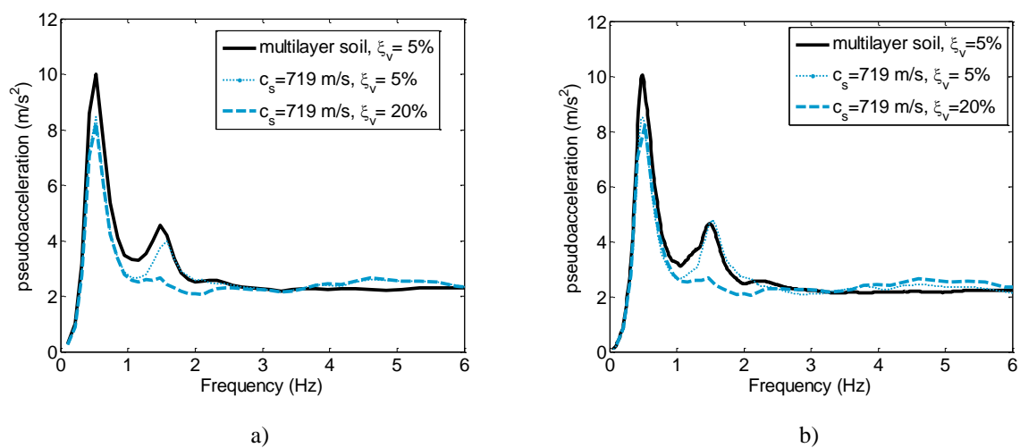
Figure 6. Spectre de plancher (5% d'amortissement), niveau inférieur du sous-sol de la structure avec isolation 3D a) modèle 3D, b) modèle axisymétrique
