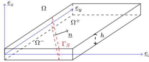
Figure 2: Surface de discontinuité \Gamma_S dans le domaine \Omega
