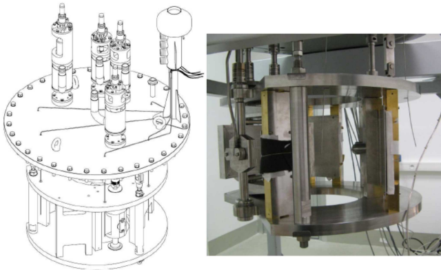
Fig. 9. MULTIREFLECTEUR mockup for telemetry sodium tests.
