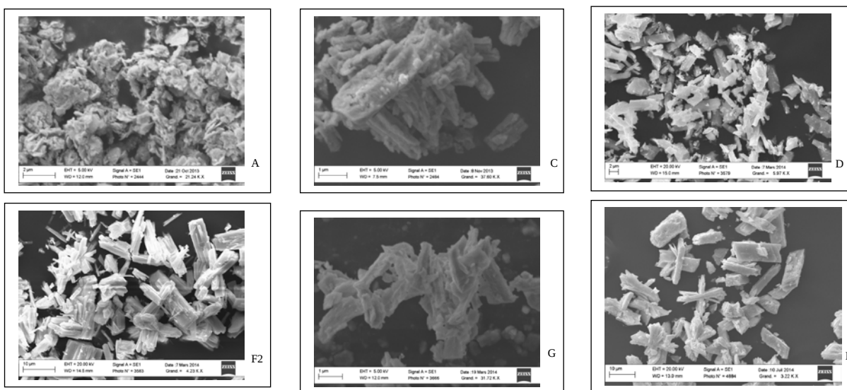
Figure 1 : Micrographies MEB des poudres d'oxydes obtenues dans les différentes synthèses
