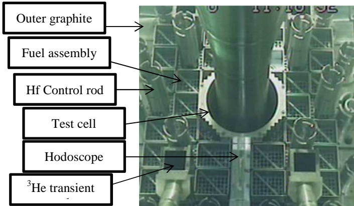
Fig. 1. CABRI core
