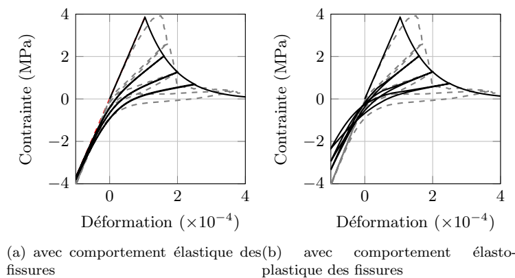
Figure 7: Réponse uni-axiale de la loi de comportement proposée sous chargement de traction cyclique.
