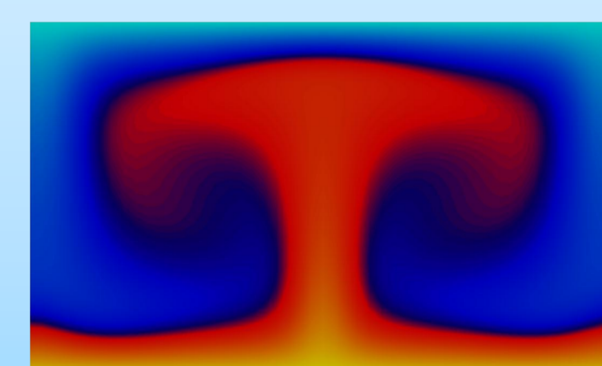
Evolution d'une stratification instable de température
