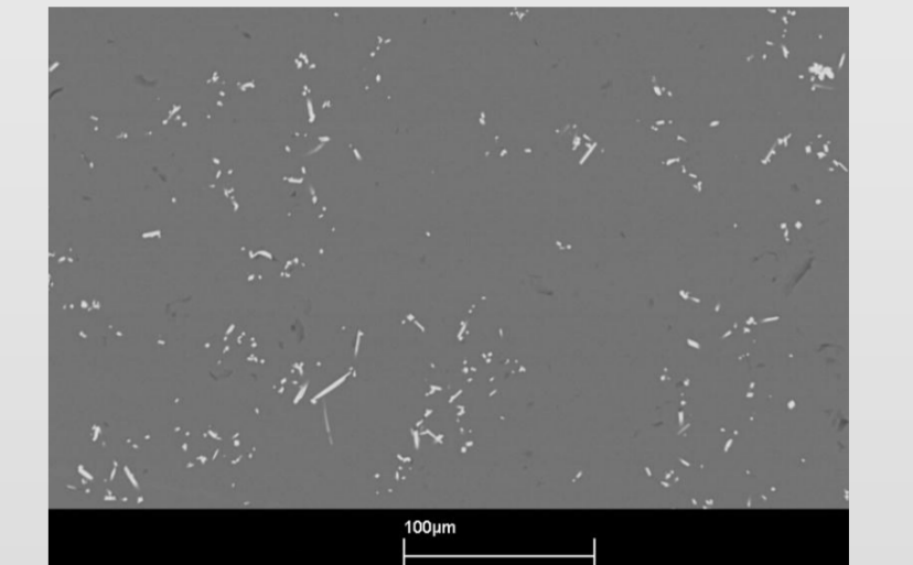
Cliché MEB de particules de dioxyde de ruthénium dans un simulant de verre nucléaire
