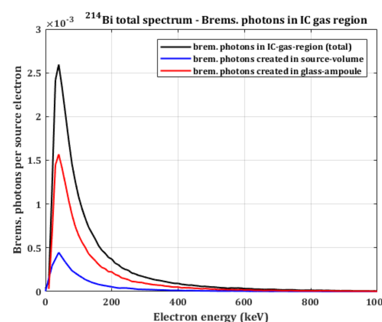
Fig. 7: Bremsstrahlung photons in IC –gas-region for ^{214}\text{Bi}
