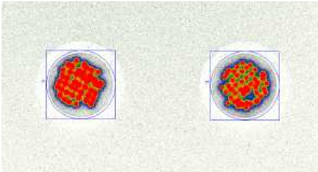
Cl-36
