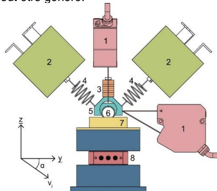
Figure 1. Diagramme du banc d'essais d'impact (1 : Capteurs de déplacement, 2 : Pots vibrants, 3 : Masse additionnelle, 4 : Ressorts de liaison, 5 : Porte-échantillon, 6 : Tube GV, 7 : Echantillon de BAV et réservoir d'eau, 8 : Capteur de force)
