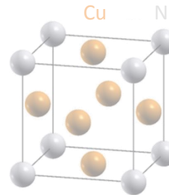
Liaisons métallique
