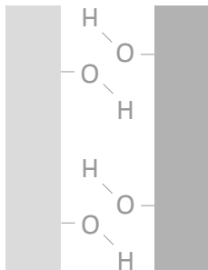
Liaisons H
