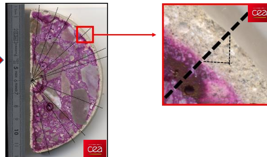
Mise en évidence d'une baisse du pH de l'eau porale après mise en contact avec l'eau
