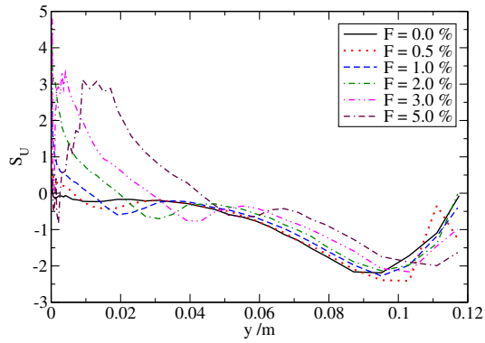
Fig. 17. Skewness factor S_U .
